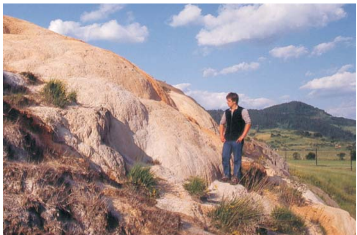
Ryc. 6. Kaskada trawertynowa we wsi Bešeňová, Słowacja
