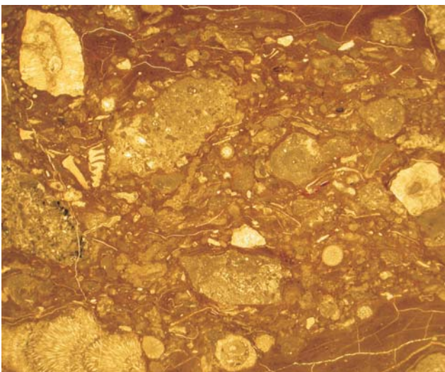
Ryc. 7. Bioklasty z turbidytów wapiennych w warstwach Partnach (głównie glony wapienne i stromatolity sinicowe), pochodzące z niszczenia facji Wetterstein, Wielkie Koryciska. Płytko cienka o szer. ok. 5 mm
