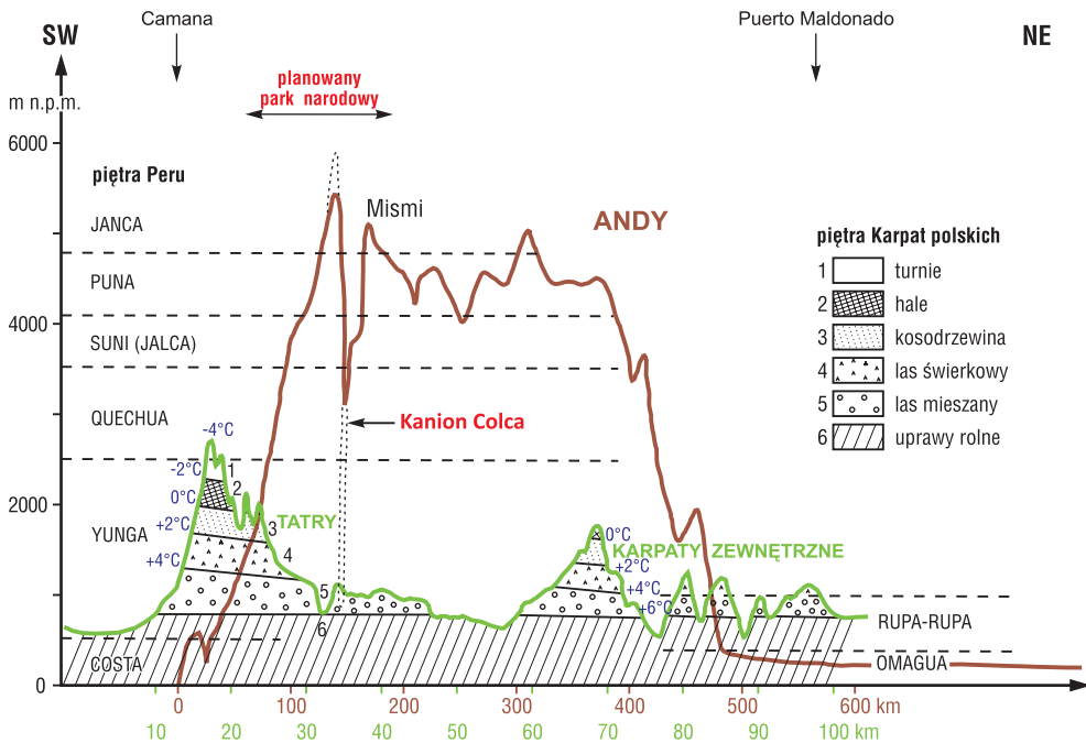
Ryc. 2. Porównanie pięter roślinno-klimatycznych w Peru (Pulgar Vidal, 1981) i w Karpatach polskich (Hess, 1965). Zwróć uwagę na różne skale poziome
