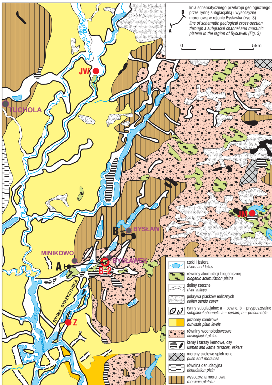
Ryc. 2. Szkic geomorfologiczny rejonu Byślawa. Opracowany na podstawie: Heliasz & Ostaficzuk (2000); Jurys & Woźniak (2006); Pikies (2006); Wieczorek & Stoiński (2006) – zmodyfikowany
