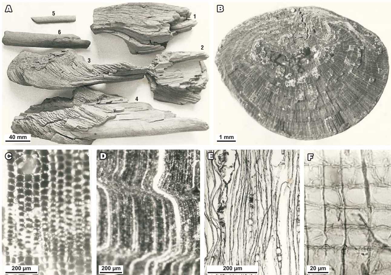
Ryc. 4. Fotografie makro- i mikroskopowe drewna sosny zwyczajnej ( Pinus sylvestris L.) z interstadiu pilicy, formacja Chojny. A – cztery fragmenty z dużych obiektów i dwie gałązki (1–4 stare pnie; 5, 6 – młode gałązki); B – przełam poprzeczny przez gałązkę (A6) z wyraźnymi asymetrycznymi przyrostami rocznymi; C – mikroskopowy przekrój poprzeczny przez drewno z kanałem żywicznym; D – poprzeczny przełam z zawichrowanym układem szeregów promieniowych wskazujący na sprasowanie drewna; E – przekrój podłużny styczny z promieniami jednorzędowymi i z promieniem wrzecionowatym zawierający poprzeczny kanał żywiczny; F – przekrój podłużny promieniowy z jamkami okienkowymi na kontakcie z komórkami miękiszowymi promienia i z cewkami promieni o ząbkowanych ścianach
