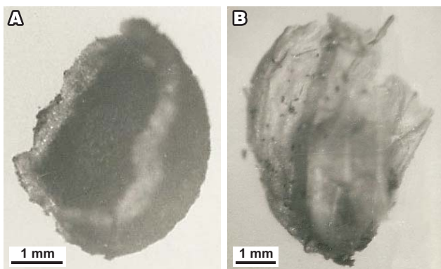
Ryc. 5. Fotografie owoców znalezionych w torfie z holocenu. A – fragment nasiona bobrka ( Menyanthes trifoliata L.); B – pecherzyk turzycy ( Carex L.)
