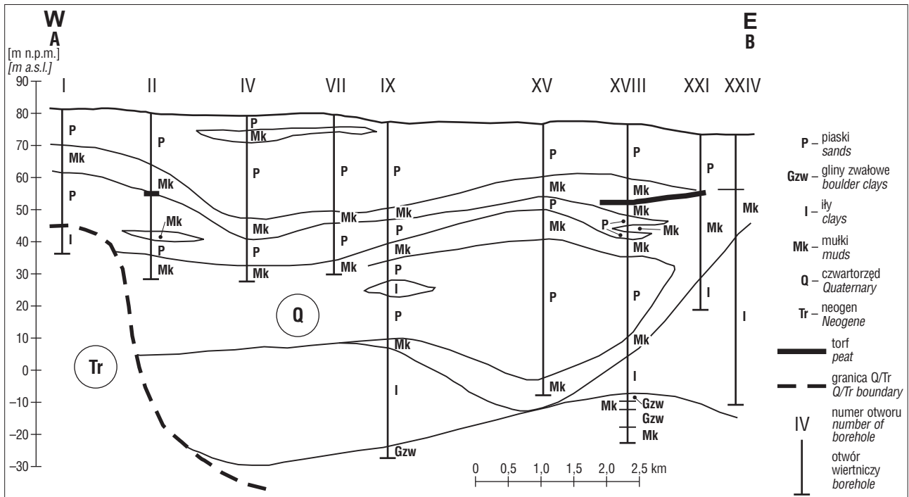
Ryc. 5. Przekrój geologiczny wzdłuż fragmentu depresji glacitektonicznej Nowej Soli (Kotowski & Kraiński, 1995). Lokalizacja przekroju – zob. ryc. 4
