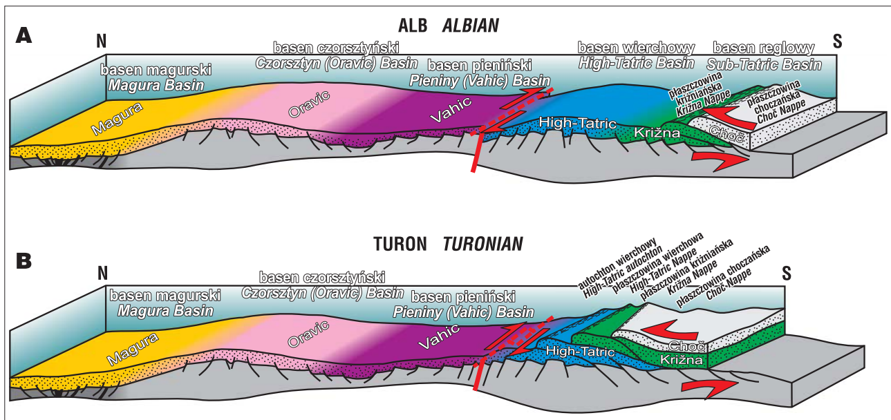
Ryc. 3. Etapy rozwoju płaszczowinowej budowy Tatr (wg Jurewicz, 2005): A – alb: odkłucie i nasunięcie płaszczowiny choczańskiej na krizniańską, odkłucie płaszczowiny krizniańskiej; B – turon: podsunięcie się trzonu krystalicznego wraz z autochtoniczną pokrywą osadową pod płaszczowinę wierchową z nasuniętą wcześniej płaszczowiną krizniańską i choczańską
