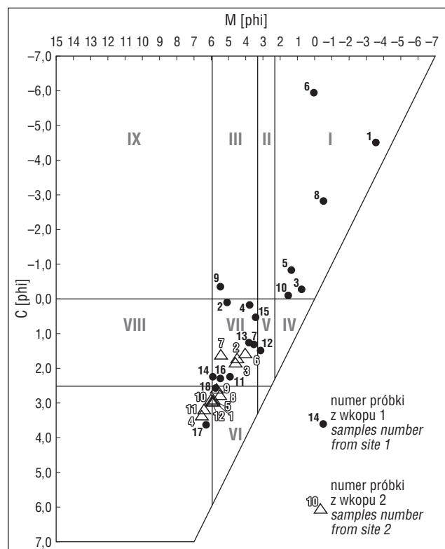
Ryc. 5. Diagram C/M dla osadów z wkopów 1 i 2
