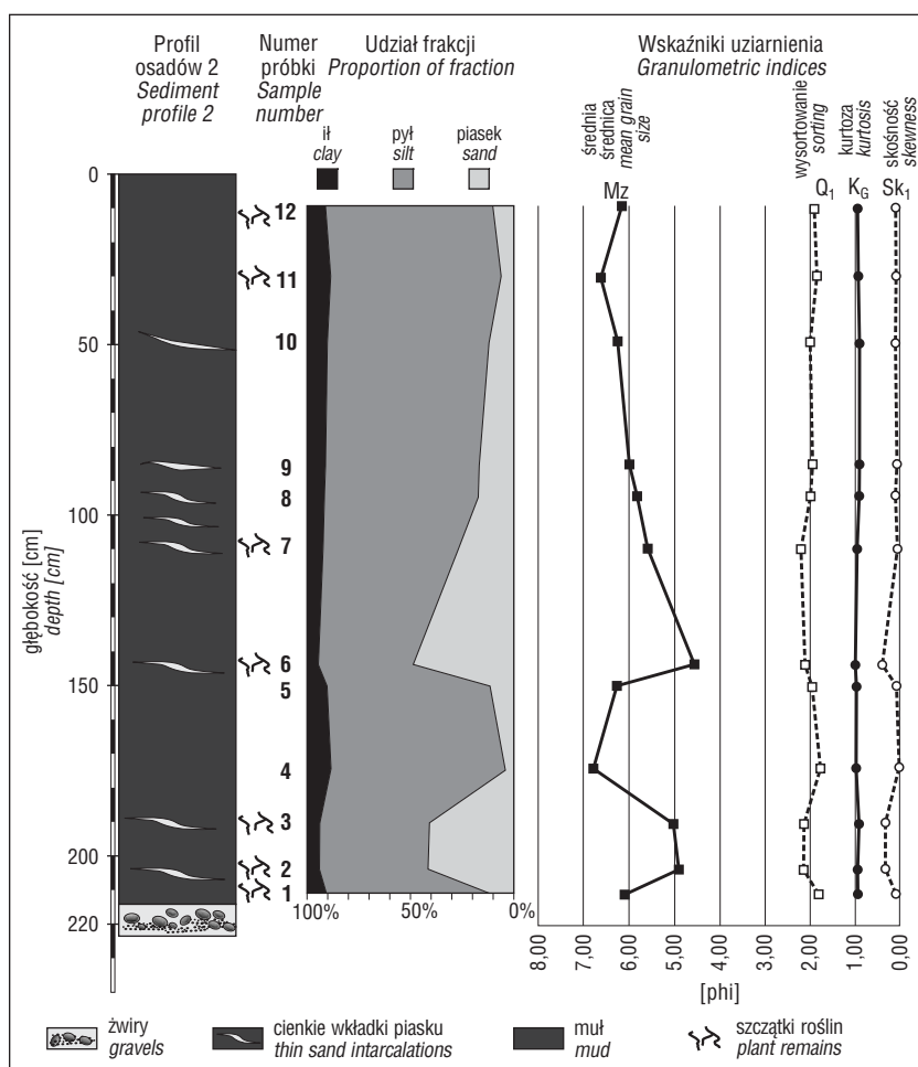
Ryc. 6. Profil osadów w kopu 2
