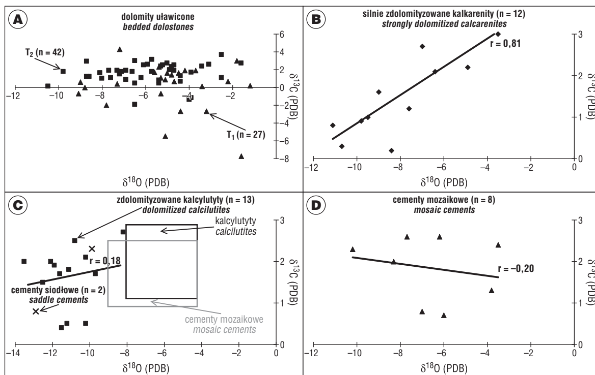
Ryc. 7. Wykresy \delta^{13}\text{C} vs \delta^{18}\text{O} dolomitów i cementów dolomitowych. Objaśnienia: r – współczynnik korelacji, n – ilość próbek. A – dolomity uławiczone (wczesnodiagenetyczne); B – silnie zdolomitowane kalkarenity; C – zdolomitowane kalcyłuty i dolomitowe cementy siodłowe; D – cementy mozaikowe
