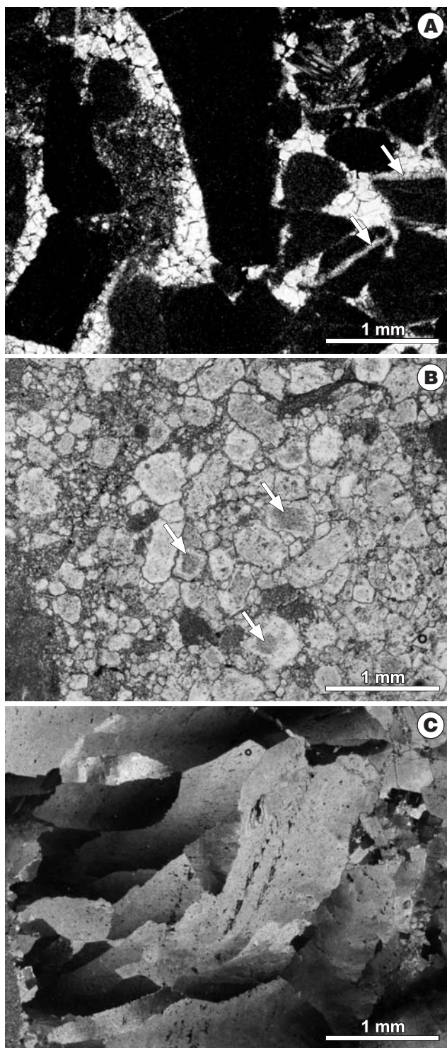
Ryc. 6. Cementy dolomitowe brekcji rozpuszczeniowo-kolapsyjnych (płytki cienkie): A – cementy drobnokrystaliczne (najstarsze odnotowane cementy, związane z wczesnym etapem pogrzebienia?; strzałki) i mozaikowe. Profil Giewontu, dolny trias; B – kryształy cementów o budowie zonalnej (strzałki) związanej z kontaminacją osadów detrytycznych. Profil Giewontu, dolny trias; C – dolomitowe cementy siodłowe (skrzyżowane nikole). Profil Giewontu, środkowy trias
