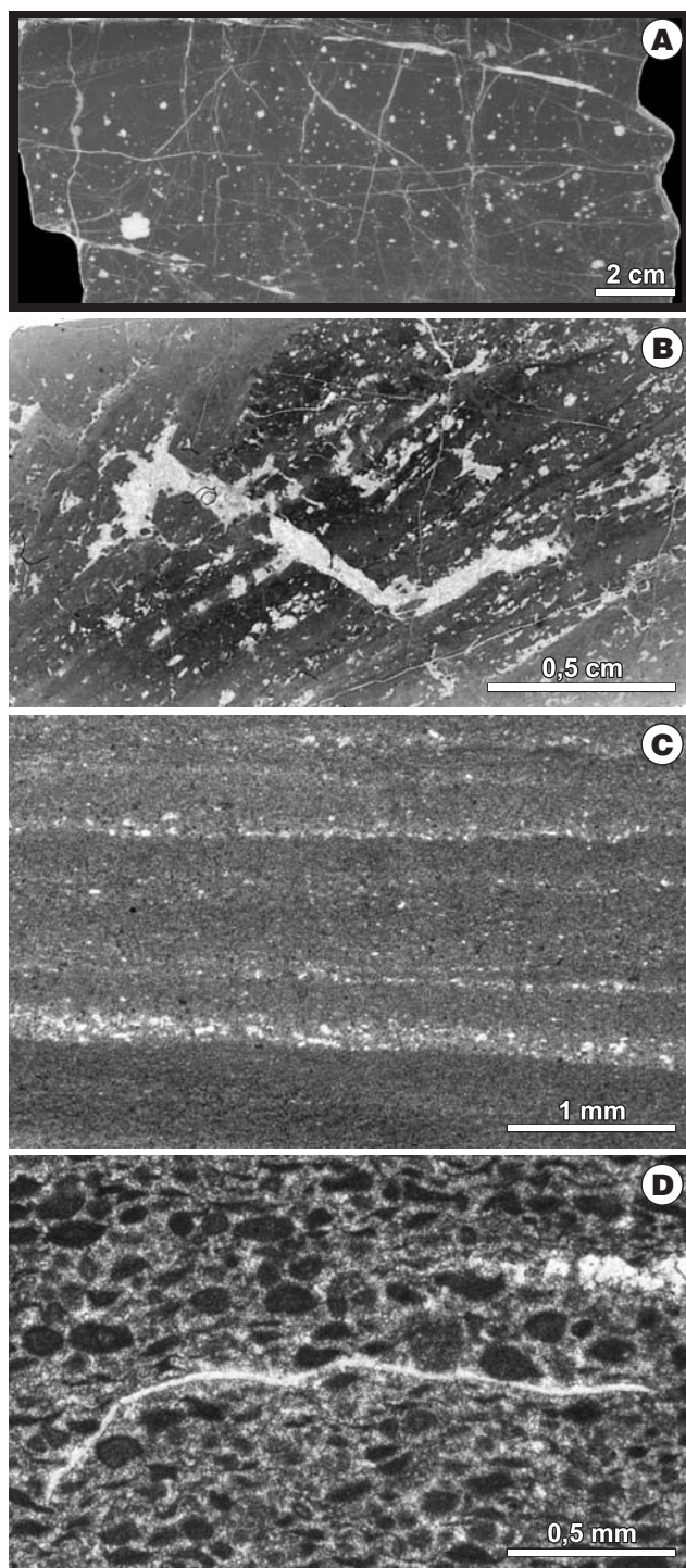
Ryc. 3. Dolomity uławiczone: A – owalne dolomitowe pseudomorfozy po siarczanach rozproszone w dololutyte (zgląd). Profil Żlebu pod Chudą Turnią, dolny trias; B – dolomit mikrobialny ze strukturami fenestralnymi; płytka cienka. Profil Giewontu, środkowy trias; C – dololutyt z laminami pyłu kwarcowego prawdopodobnie pochodzenia eolicznego (płytko cienka). Profil Iwanowskiego Potoku, dolny trias; D – pakston peloidowo-intraklastowy (płytko cienka). Profil Giewontu, dolny trias
