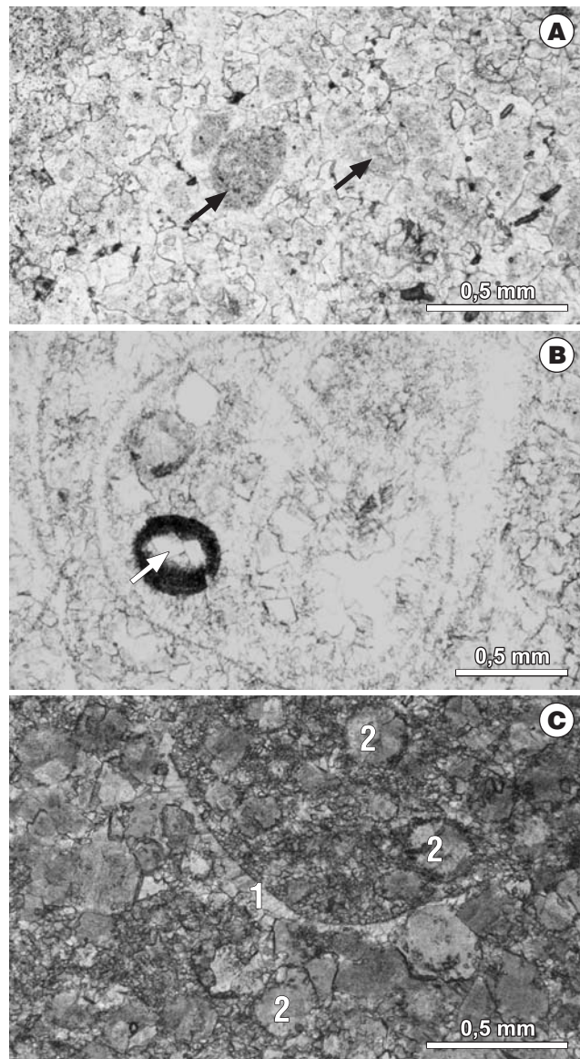
Ryc. 4. Zdolomityzowane kalkarenity triasu środkowego (płytki cienkie): A – zdolomityzowany grejnston peloidowo-oidalowy? Pierwotne allochemy (peloidy) zachowane jako „duchy” (strzałki). Profil Giewontu; B – pakston ślimakowo-oidalowy. We wnętrzu zmikrytyzowanego ooidu euhedralne kryształy dolomitu (strzałka) – dowód moldycznej porowatości. Profil Kominiarskiego Wierchu; C – całkowicie zdolomityzowany pakston ooidalno-małżowy (skrzyżowane nikle). Zachowane obrysy komponentów małża (1) i ooidów (2) wypełnione przez krystaliczny dolomit. Profil Kominiarskiego Wierchu
