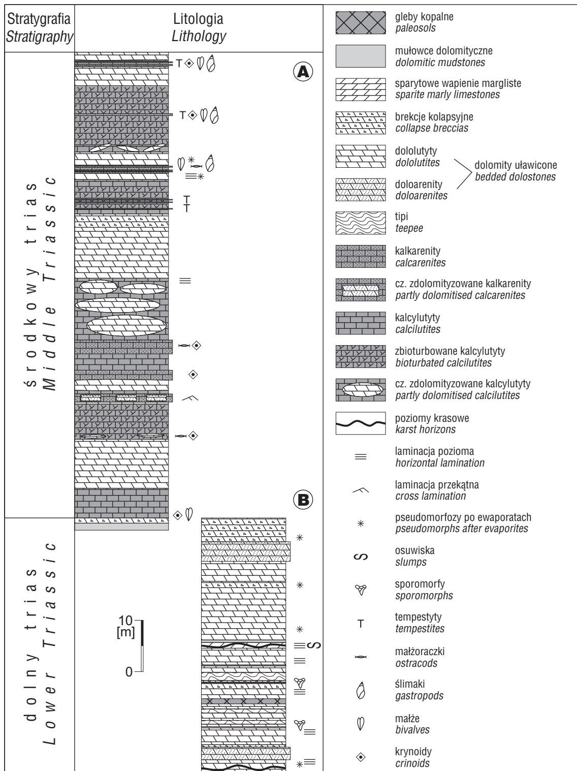
Ryc. 2. Przykładowe profile utworów węglanowych triasu dolnego i środkowego serii wierzchowej Tatr Zachodnich (płaszczyzna Czerwonych Wierchów): A – profil Koziego Grzbietu; B – profil Żlebu pod Chudą Turnią Fig. 2. Exemplified sections of the Lower and Middle Triassic carbonates of the High-Tatric series (Czerwone Wierchy Nappe): A – Kozi Grzbiet section; B – Żleb pod Chudą Turnią section
