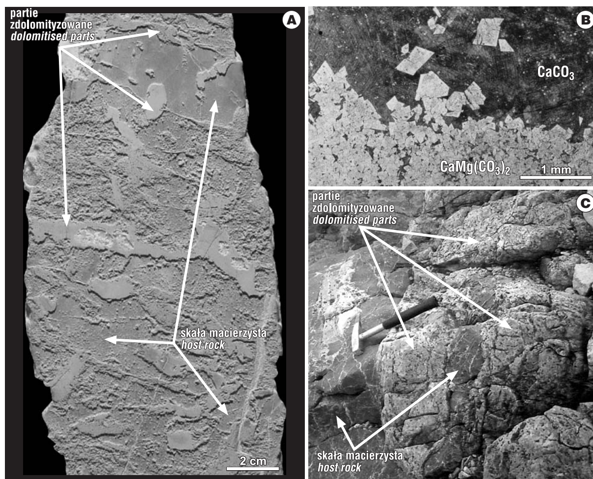
Ryc. 5. Zdolomityzowane kalkylutytry triasu środkowego: A – selektywnie zdolomityzowany kalkylutyt ze strukturami bioturbacyjnymi (powierzchnia zglądu trawiona kwasem mrówkowym). Profil Kominiarskiego Wierchu; B – szczegóły A. Struktury bioturbacyjne wypełnione euhedralnymi kryształami dolomitu. Ciemne pole (w rzeczywistości czerwone) – \text{CaCO}_3 , białe pole – \text{CaMg}(\text{CO}_3)_2 , płytka cienka barwiona roztworem czerwieni alizarynowej S + żelazicyjanu potasu; C – gniazdowa dolomityzacja w obrębie kalkylutytów. Profil Giewontu
