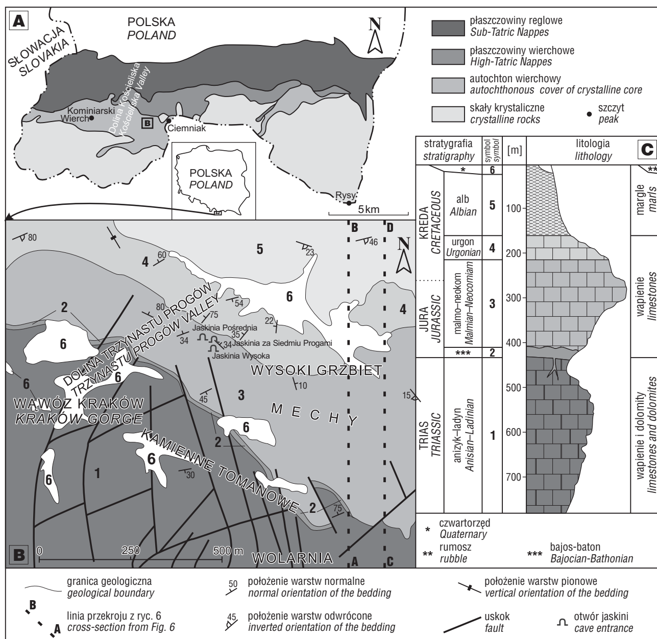
Ryc. 1. A – obszar badań na tle głównych jednostek tektonicznych Tatr (wg Bac-Moszaszwili i in., 1979); B – powierzchniowa budowa geologiczna obszaru badań (Piotrowski, 1978; Piotrowska i in., 2008; zmienione); C – profil litostratigraficzny serii Wąwozu Kraków (wg Kotańskiego, 1961; zmienione)
