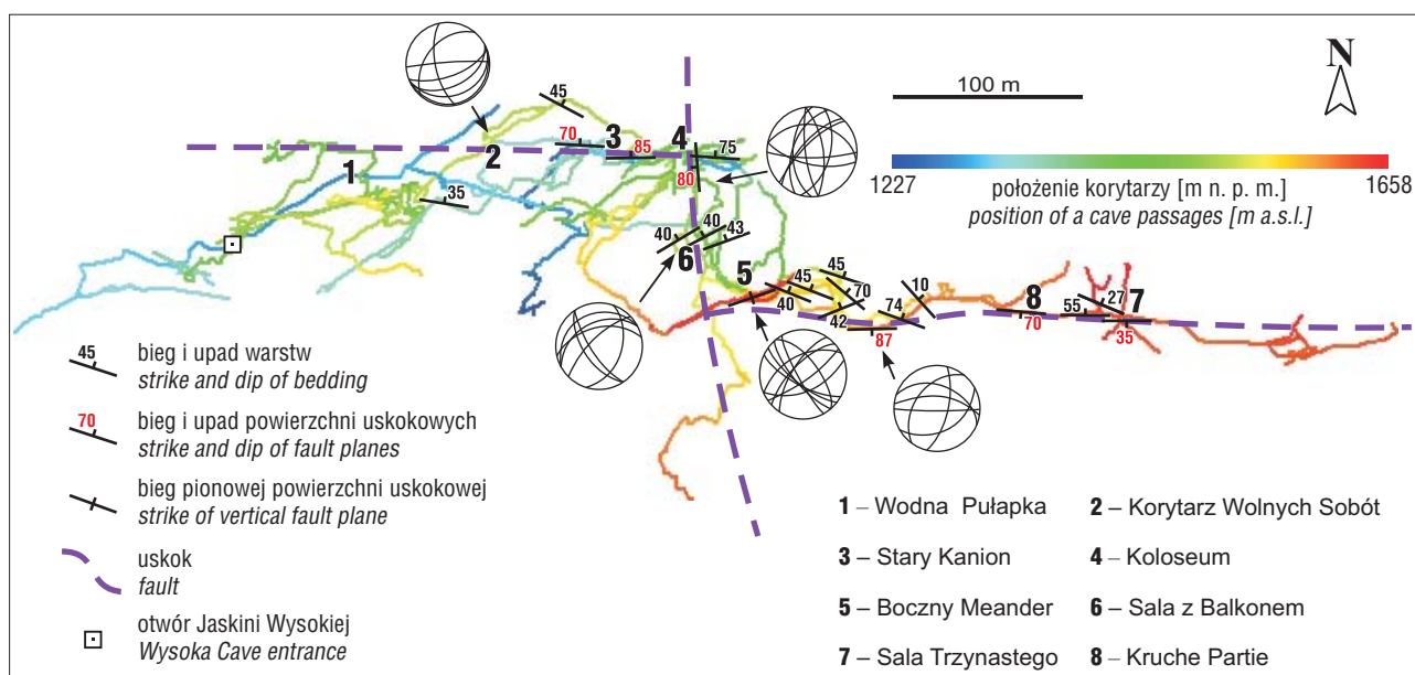
Ryc. 3. Plan strukturalny systemu jaskiniowego Wysoka – Za Siedmiu Progami (diagramy spękań na półkuli dolnej)
