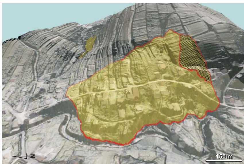
Ryc. 5. A – Porównanie zasięgu osuwiska w Łańnicy na tle ortofotomapy; B – Przykład uszkodzonego budynku mieszkalnego w Łańnicy Fig. 5. A – Comparing coverage of landslide in Łańnica on the background orthophoto; B – An example of the destroyed building in Łańnica
