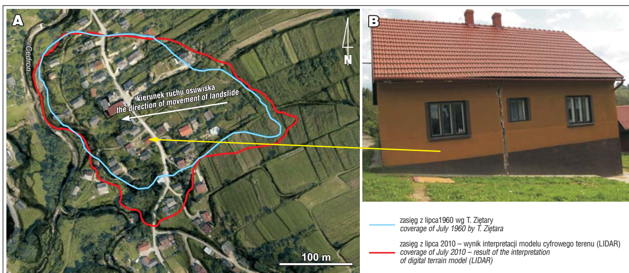
Ryc. 5. A – Porównanie zasięgu osuwiska w Łańnicy na tle ortofotomapy; B – Przykład uszkodzonego budynku mieszkalnego w Łańnicy Fig. 5. A – Comparing coverage of landslide in Łańnica on the background orthophoto; B – An example of the destroyed building in Łańnica
