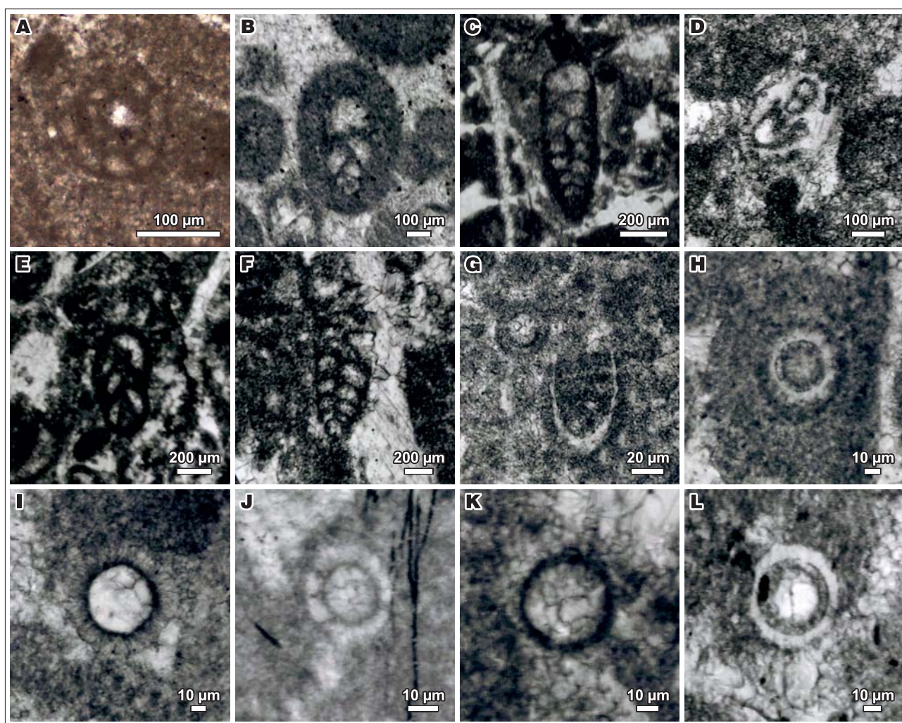
Ryc. 4. Mikroskamieniałości z wapieni profilu Niedźwiedź. A – Debarina hahounerensis Fourcade, Raoult et Vila, (przekrój poprzeczny), Ni1; B – Haghimashella arcuata Haeusler, (przekrój podłużny), Ni68; C – Protomarssonella kummi (Zedler), (przekrój podłużny), Ni21; D – Protopenereplis ultragranulata (Gorbatchik), (przekrój poprzeczny), Ni46; E – Textulariopsis jurassica (Guembel), (przekrój podłużny), Ni46; F – Uvigerinammina uvigeriniformis (Seibold et Seibold), (przekrój podłużny), Ni81; G – Tintinnopsella carpathica (Murgeanu et Filipescu), Ni61; H – Colomisphaera tenuis (Nagy), Ni65; I – Colomisphaera varia Řechanek, Ni34; J – Colomisphaera lucida Borza Ni90; K – Cadosina minuta Borza, Ni61; L – Parastomiosphaera malmica (Borza), Ni92
