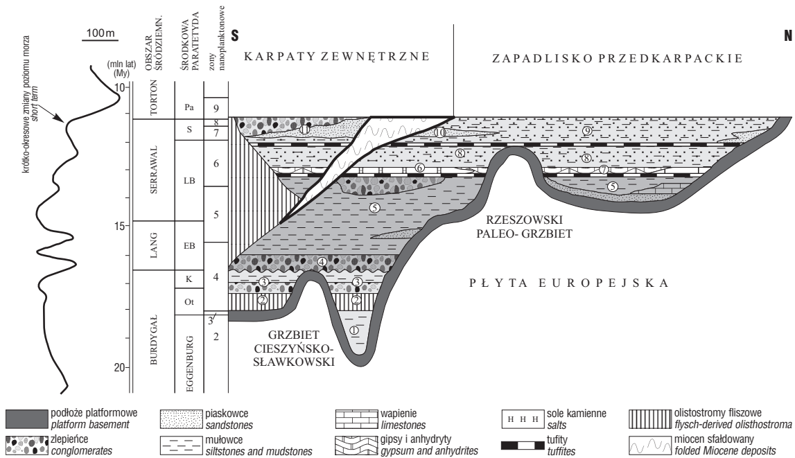
Ryc. 4. Schemat litostratigraficzny osadów miocenijskich zapadliska przedkarpackiego (według Oszczycki, 1999 — uzupełniony); jednostki litostratigraficzne: 1 — formacja zebrzydowicka, 2 — formacja suska oraz ogniwo z Zamarskich, 3 — formacja stryszawska, 4 — zlepieńce dębowieckie, 5 — formacja skawińska i warstwy baranowskie, 6 — formacja wielicka, 7 — formacja z Krzyżanowic, 8 — warstwy chodenickie, 9 — warstwy grabowieckie i krakowieckie, 10 — piaski bogucickie, 11 — warstwy z Nockowej i formacja z Beli; Ot — Ottngang, K — Karpat, EB — wczesny baden, LB — późny baden, S — sarmat, Pa — panon
