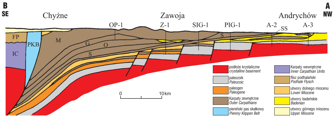
Ryc. 2. Przekrój geologiczny (A–B) Andrychów–Chyżne (usytuowanie na ryc. 1B) według Oszczyпки (1997, uzupełniony)
