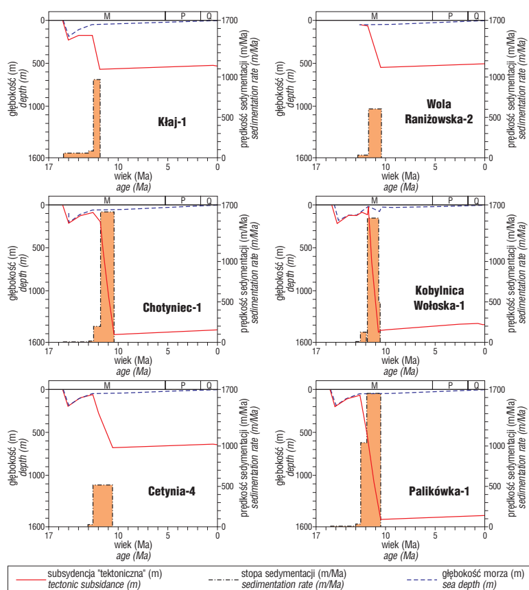
Ryc. 5. Diagramy subsydemcji „tektonicznej” w wybranych wierceniach środkowej i wschodniej części zapadliska przedkarpackiego (Oszczypko, 1999)
