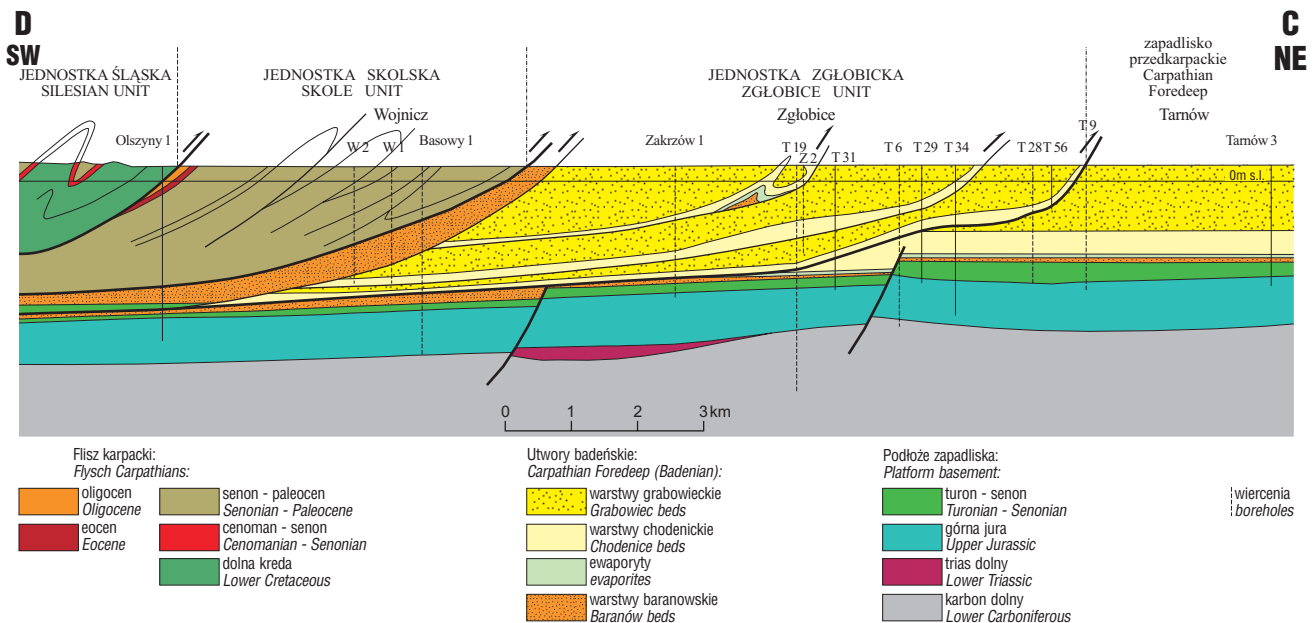
Ryc. 3. Przekrój geologiczny (C–D) Olszyny–Tarnów (usytuowanie na ryc. 1B) według Oszczyпки (1999)
