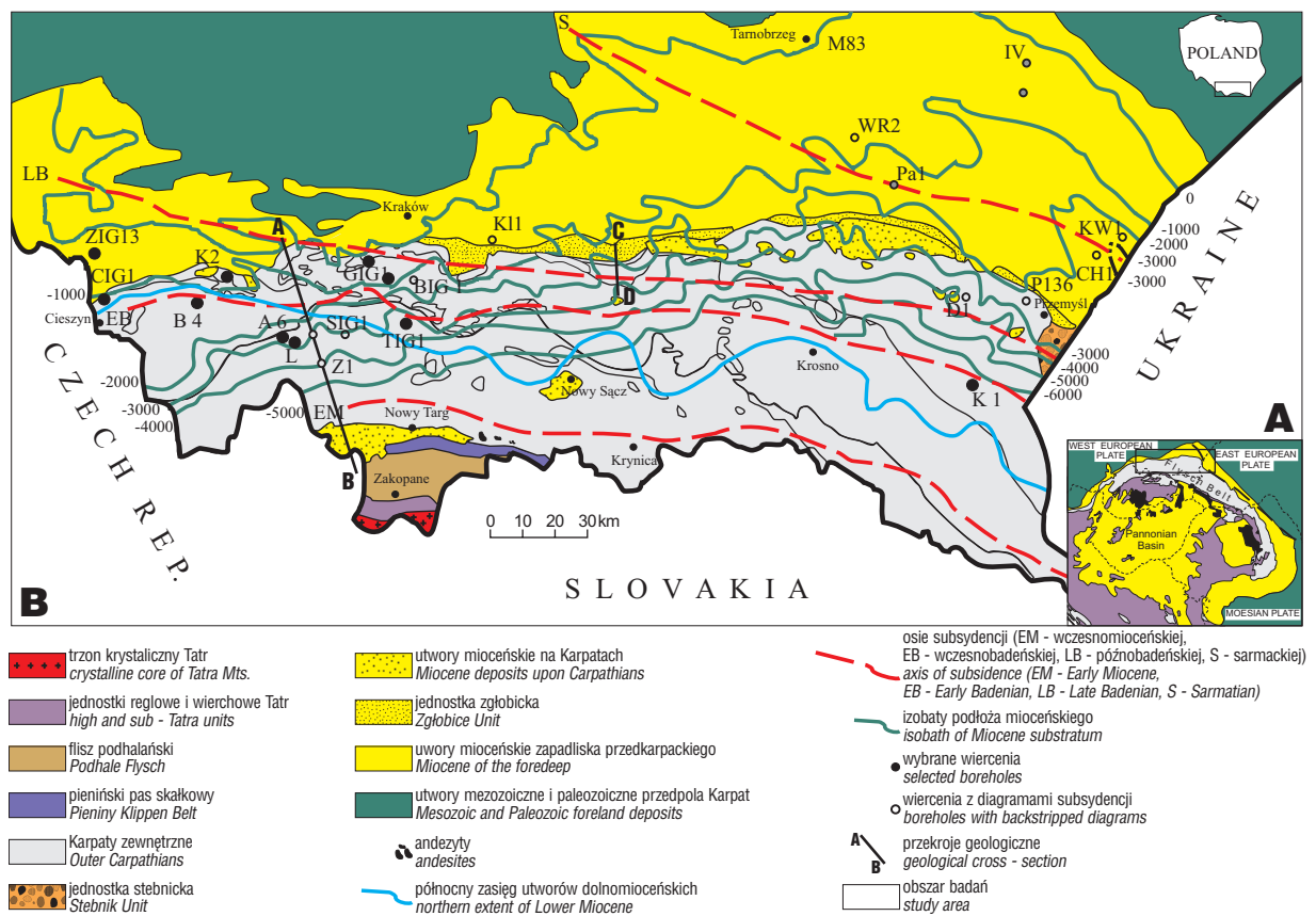
Ryc. 1. A — Usytuowanie polskiej części zapadliska przedkarpackiego w obszarze karpacko-panońskim. B — Szkic tektoniczny polskiej części Karpat i zapadliska przedkarpackiego (według Oszczytko, 1997, uzupełniony) Fig. 1. A — Location of the Polish Carpathian Foredeep in the Carpathian–Pannonian region. B — Sketch–map of the Polish Carpathians and their foredeep (after Oszczytko, 1997 supplemented)
