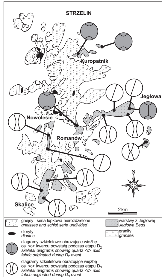
Ryc. 12. Mapa więźby osi c kwarcu w obrębie warstw z Jęglowej Fig. 12. Map of quartz c axis fabrics in the Jęglowa beds
