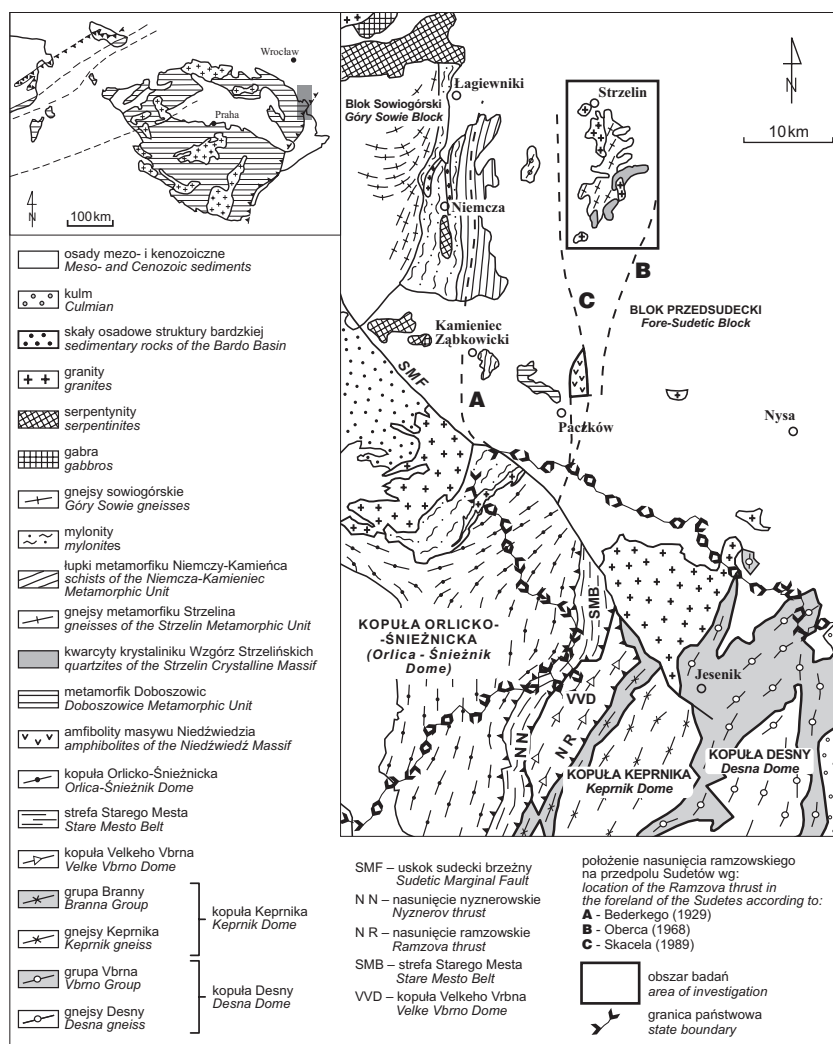
Ryc. 1. Położenie obszaru badań na tle budowy geologicznej regionu; wkładka obrazuje położenie obszaru badań na mapie Polski (wg Puziewicz i in., 1999) Fig. 1. Regional setting of the study area; the inset shows location of the study area on the map of Poland after Puziewicz et al. (1999)
