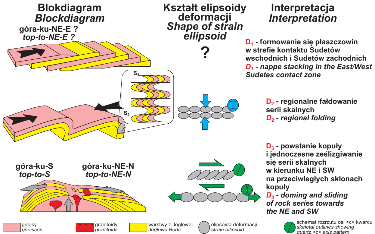
Ryc. 13. Blokdiagram przedstawiający schemat ewolucji tektonicznej skał warstw z Jęglowej w krystaliniku Wzgórz Strzelińskich Fig. 13. Blockdiagram showing scheme of tectonic evolution of the Jęglowej beds in the Strzelin crystalline massif
