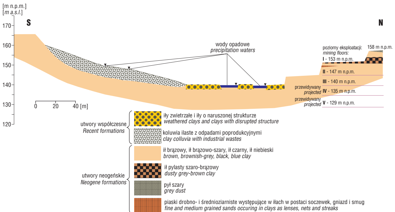
Ryc. 3. Przekrój geologiczny przez odkrywkę iłów w Budach Mszczonowskich
