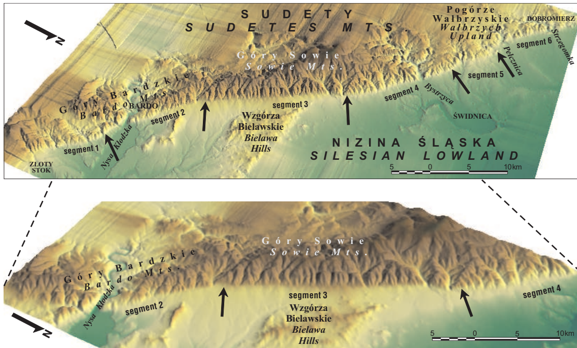
Ryc. 4. Cyfrowy model terenu sudeckiego uskoku brzeźnego — widok ze wschodu. Dwukrotne przewyższenie skali pionowej Fig. 4. Digital elevation model of the Sudetic Marginal Fault — detailed view from the east. Vertical exaggeration 2 x
