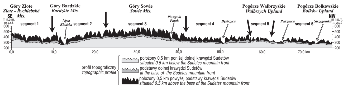
Ryc. 6. Profile podłużne badanego odcinka podnóża czoła masywu górskiego Sudetów
