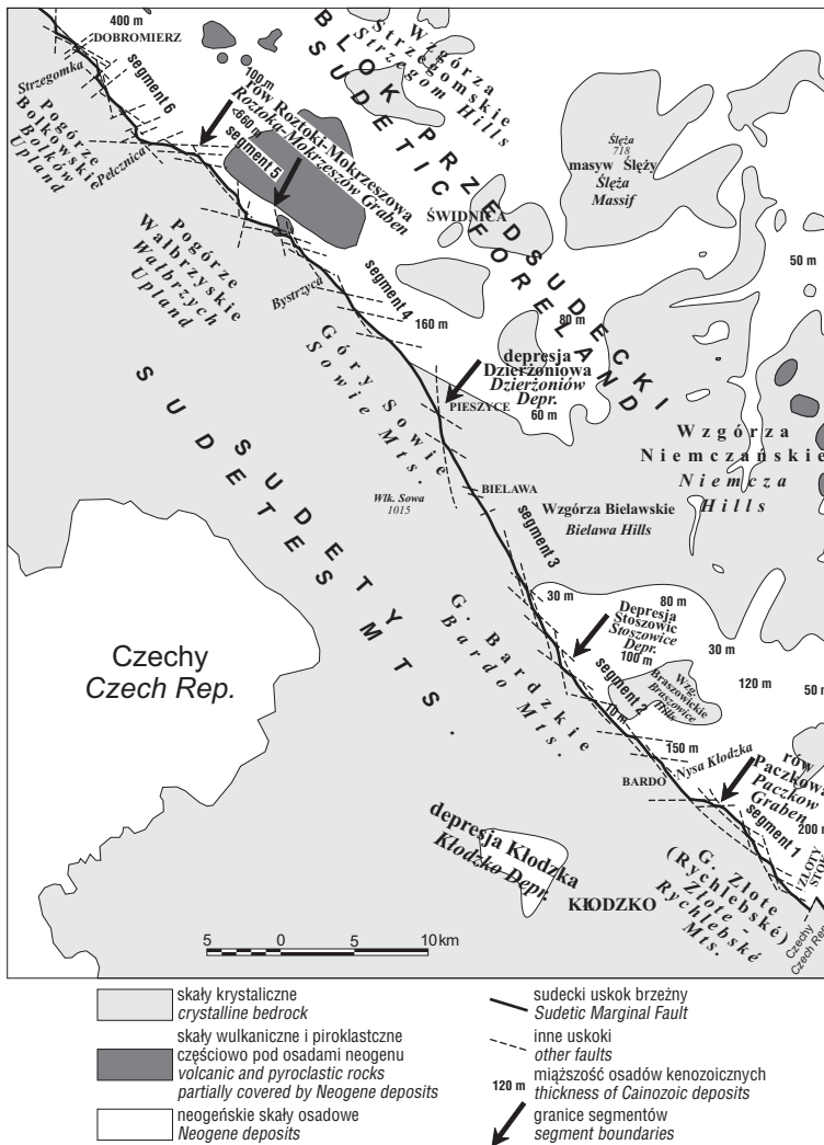
Ryc. 2. Drobne uskoki w strefie sudeckiego uskoku brzeżnego, interpretowane na podstawie cyfrowego modelu terenu i układu topolineamentów Fig. 2. Small-scale faults in the Sudetic Marginal Fault zone, interpreted from digital elevation model and topolineament pattern
