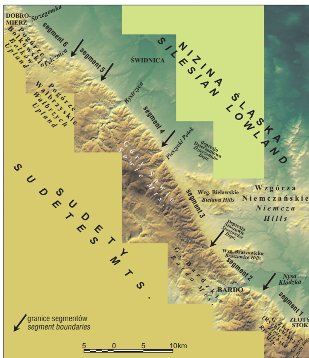
Ryc. 3. Cyfrowy model terenu sudeckiego uskoku brzeżnego — widok ogólny badanego odcinka Fig. 3. Digital elevation model of the Sudetic Marginal Fault — general view of the fault stretch studied
