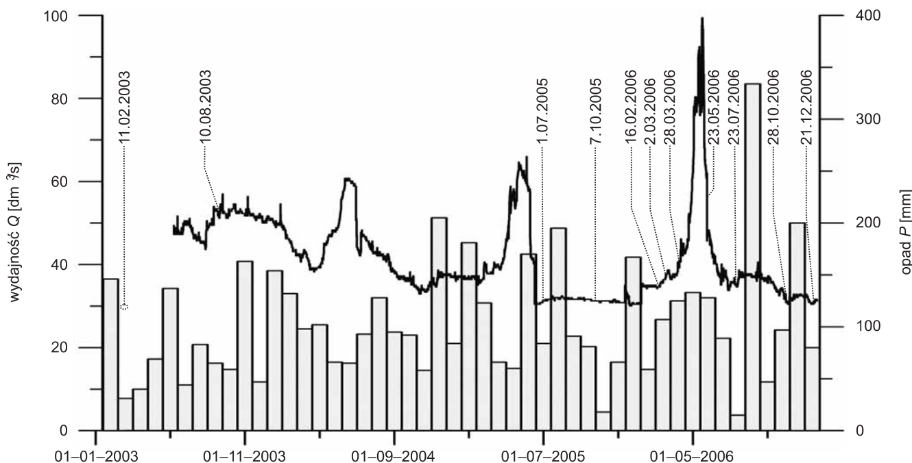
Fig. 2. Wydajność strefy źródłiskowej w Zieléncu (maj 2003–grudzień 2006) na tle wysokości miesięcznych sum opadów (styczeń 2003–grudzień 2006) z zaznaczonymi miejscami opróbowania (poza okresem objętym na wykresie, próbki pobrano 20.02.2007; 05.05.2007; 06.07.2007; 13.10.2007)
