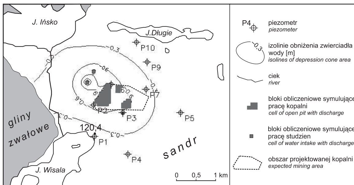
Fig. 6. Symulacja C – mapa wypadkowego leja depresji poziomu sandrowego dla warunków maksymalnego poboru wody z istniejących studzien i 20-krotnie zawyżonej wartości ubytku wody wywołanej pracą kopalni
