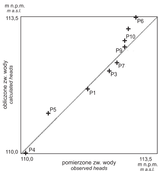
Fig. 4. Porównanie pomierzonego i obliczonego położenia zwierciadła wody w piezometrach
