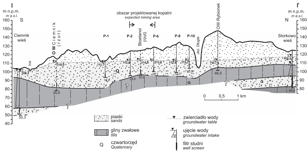
Fig. 2. Przekrój hydrogeologiczny
