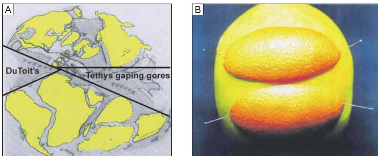
Fig. 15 A. Du Toit's Tethys gaping gores.
