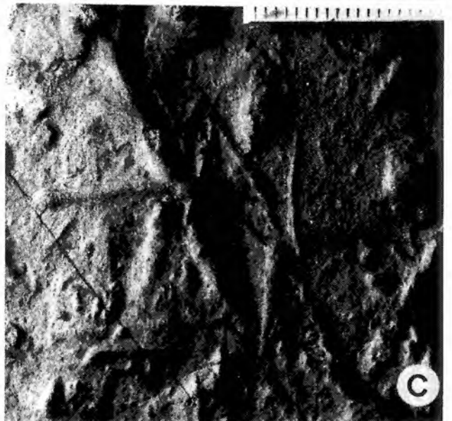
Fig. 5. Arthrophyucus strictus Książkiewicz (arrowed) and Arthrophyucus tenuis (Książkiewicz). A-C. Details of Fig. 4. Scales in mm
