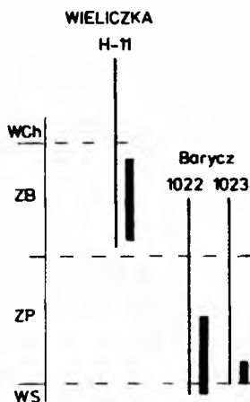
Fig. 9. Pozycja stratygraficzna opróbowanych fragmentów otworów H-11, 1022/86, 1023/85. WS — warstwy skawinińskie; ZP — złożo pokładowe; ZB — złożo bryłowe; WCh — warstwy chodenickie; o — opróbowanie
