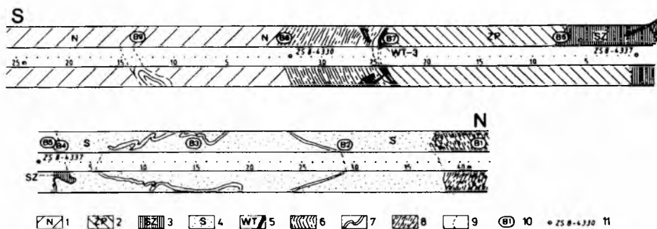
Fig. 8. Profil odcisów poprzeczni Barycz (poziom VIII) wg M. Furowej (archiwum kopalni). 1 — sól najstarsza; 2 — zespół soli zielonych pokładowych; 3 — sole szybkowe; 4 — sole spizowe; 5 — wkładka tuftowa; 6 — piaskowiec „podsolny”; 7 — sól włóknista; 8 — iłowiec stropowy; 9 — granice kompleksów; 10 — miejsca pobrania próbek; 11 — punkty geodezyjne
