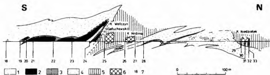
Fig. 2. Profil poprzeczni Walczyn (poziom III) wg Gawła (1962). 1 — piaskowiec „podsolny”; 2 — sole zielone pokładowe; 3 — sól szybikowa; 4 — sole spizowe; 5 — otwory bezsolne złoża bryłowego; 6 — bryły soli w złożu bryłowym; 7 — miejsca pobrania prób; K — komora
