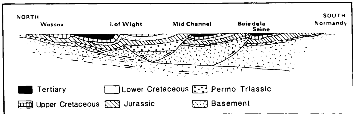
Fig. 13. Hypothetical cross section of the English Channel from Wessex to the Baie de la Seine Fig. 13. Hipotetyczny przekrój przez Kanał La Manche między Wessex a Baine de la Seine
