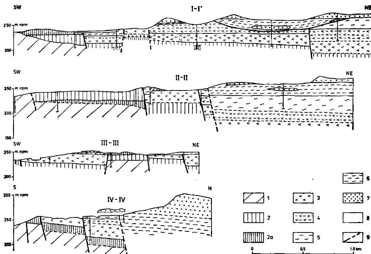
Fig. 2. Przekroje geologiczne ilustrujące budowę zachodniej części zapadliska połanieckiego. 1 — kreda, 2 — warstwy podgipsowe, 2a — wapień litotamniowe, 3 — gipsy szklicowe i szkieletowe, 4 — gipsy płytkowe, 5 — warstwy pektenowe, 6 — warstwy krakowieckie (facja ilasta), 7 — sarmat detrytyczny, 8 — czwartorzęd, 9 — uskoki
