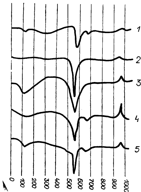
Fig. 3. Termogramy minerałów ilastych poskaleniowych
