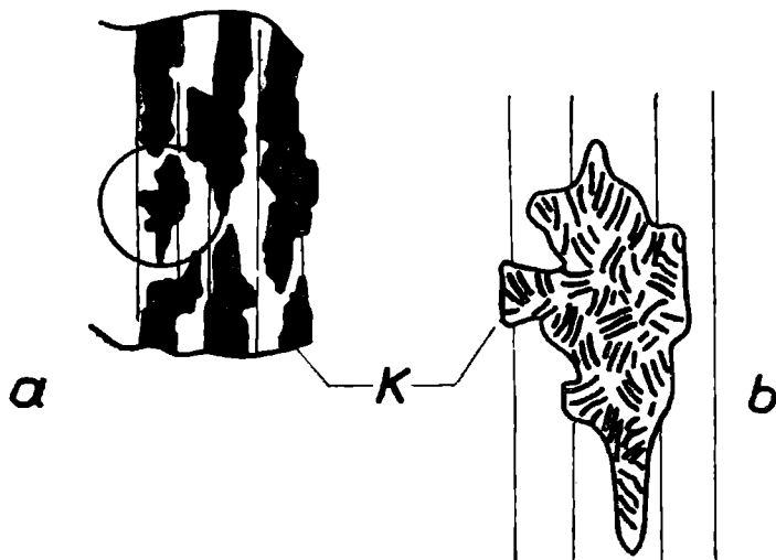
Fig. 6a. Schematyczny rysunek kaolinizacji skalenia wzdłuż łupliwości; przekrój ac , powiększenie około 500X
