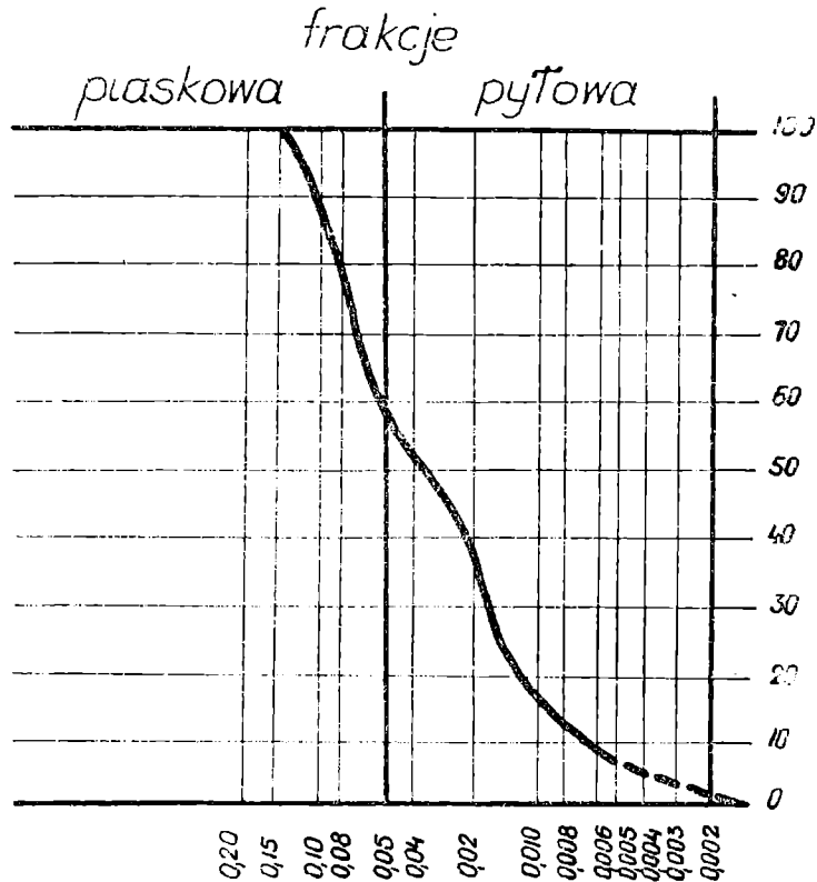
Fig. 4. Uziarnienie kaolinitu
