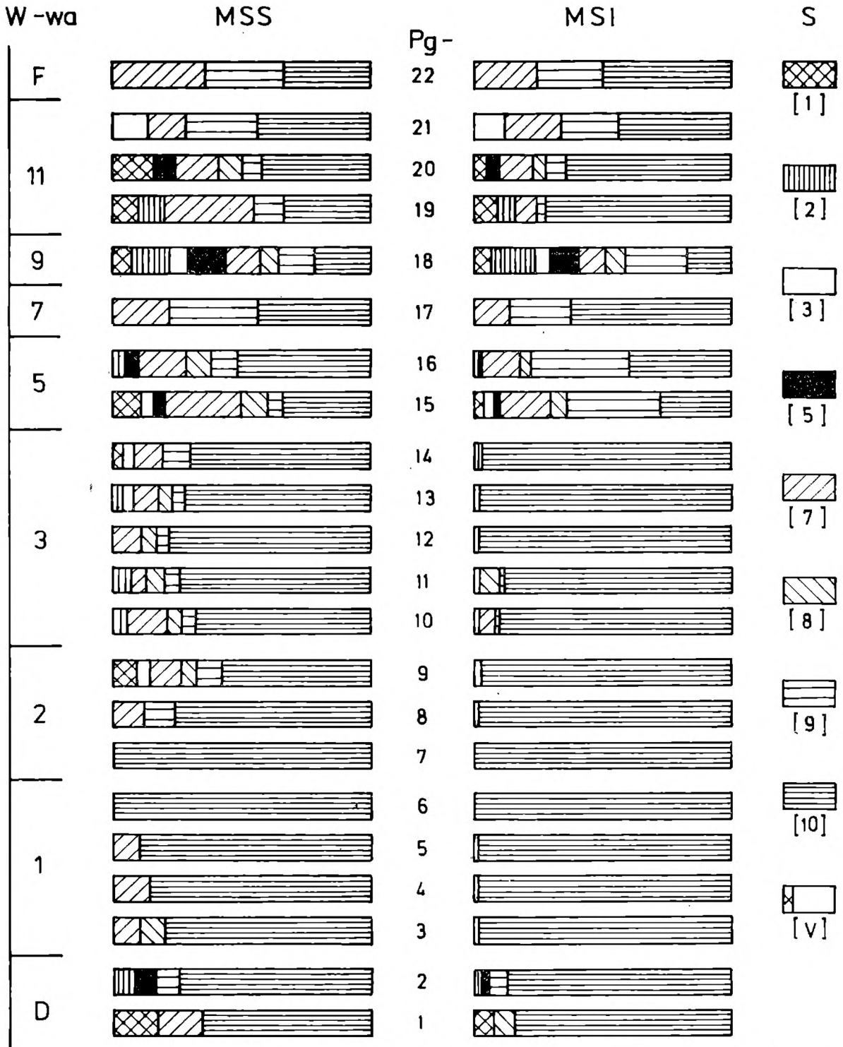
Fig. 5. Spektra malakofauny z Podgrodzia; MSS — malakospektra gatunkowe, MSI — malakospektra osobnicze, 1—10 — symbole grup ekologicznych (wg V. Ložka, 1964), v — różne grupy ekologiczne (akcesorycznie reprezentowane)
