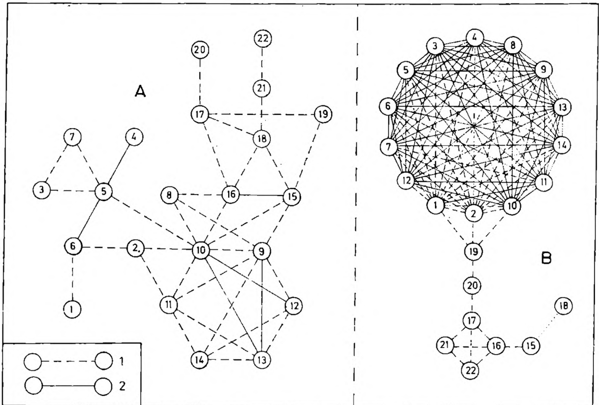
Fig. 4. Struktury taksonomiczne zespołów malakofauny; 1—22 — numery próbek, A — diagram wg metody jakościowej (wzór Steinhausa), B — diagram wg ilościowej metody różnic przeciętnych, 1 — połączenie II-go stopnia (słabe), 2 — połączenie I-go stopnia (silne)
