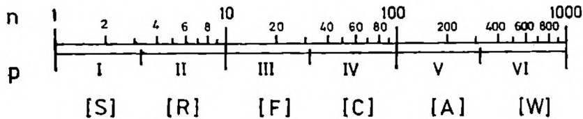
Fig. 1. Logarytmiczna skala symboli częstotliwości fauny kopalnej (określenia półilościowe); n — liczba okazów, p — symbole określeń półilościowych (liczbowe i literowe)
