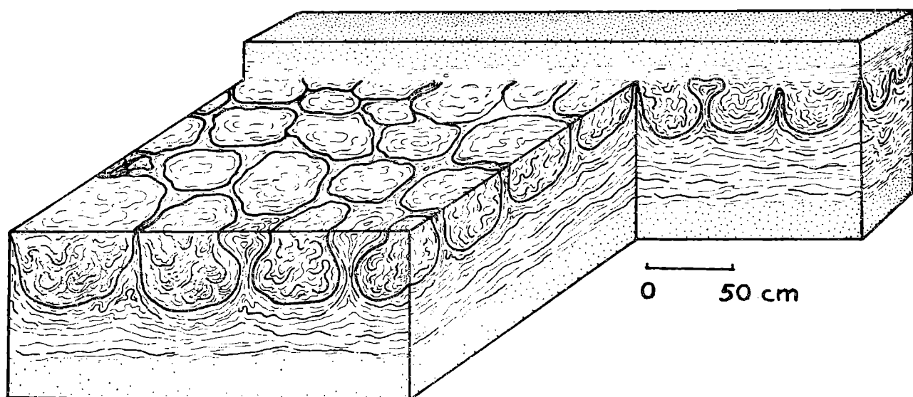
Fig. 1. Wzór przestrzenny struktur konwolucyjnych w dwuczłonowej ławicy utworzony przy całkowitym braku przemieszczenia między członami. k_1 \ll k_2 ( k_1 — lepkość kinematyczna górnego członu z riplemarkami, k_2 — lepkość kinematyczna dolnego, równoległe laminowanego członu)
