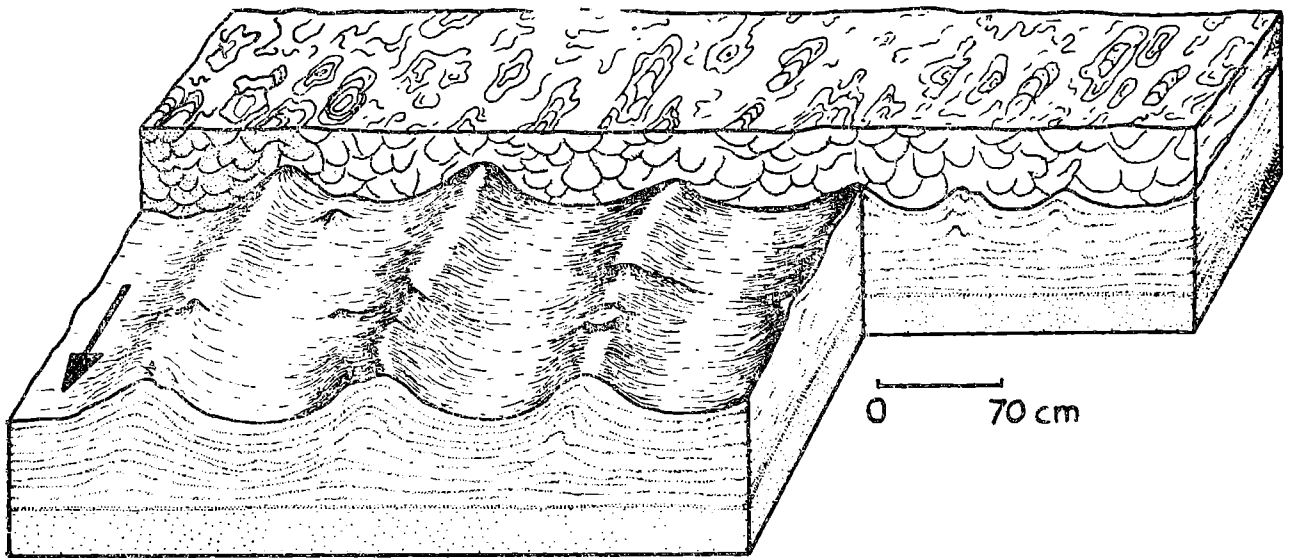
Fig. 2. Wzór przestrzenny struktur konwolutnych w dwudzielnej ławicy przy niewielkim przesunięciu poziomym między członami. k_1 \approx k_2 . Górny człon złożony ze zmaczek piaszczystych, dolny — laminowany równoległe. Porównaj z fig. 2 Tabl. XXXVII
