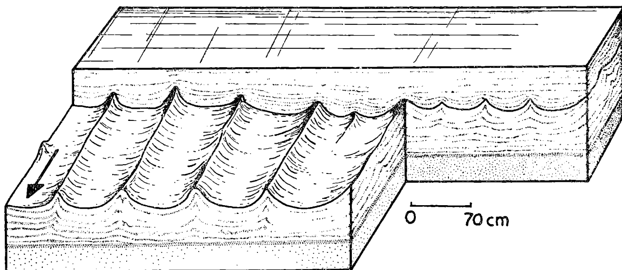
Fig. 4. Wzór przestrzenny konwolucji w warunkach jak na fig. 3. Obydwa człony równoległe laminowane. k_1 \ll k_2
