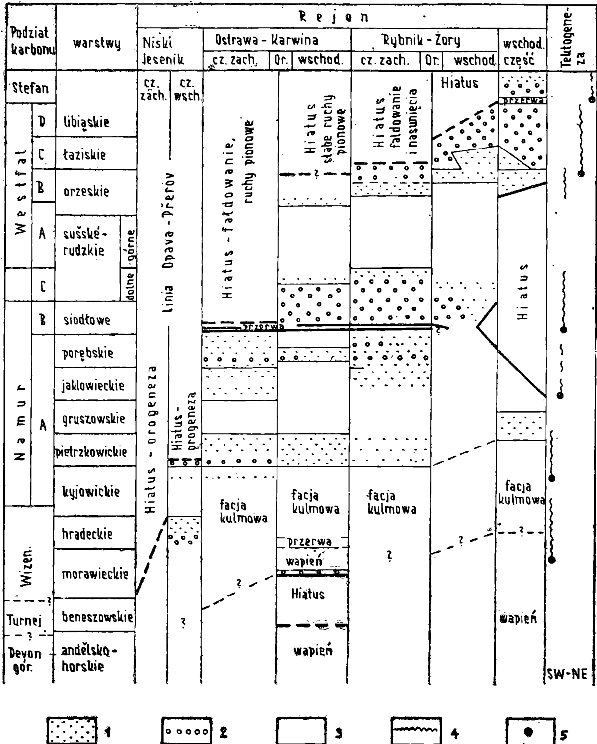
Fig. 2. Schematyczne przedstawienie związku tektogenezy, hiatusów i typów sedymencji. 1 — niewyraźne osiadanie synorogeniczne; 2 — wyraźne osiadanie synorogeniczne; 3 — sedymentacja „anorogeniczna”; 4 — ciągłość fałdowań na zapleczu; 5 — początek przesuwania się zbiornika z SW na NE
