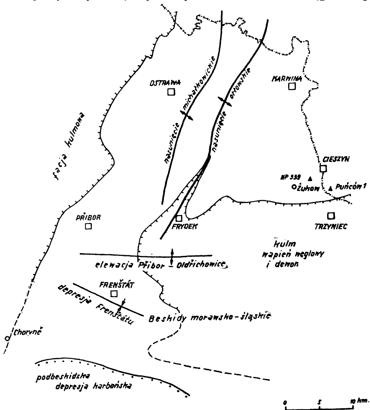
Fig. 1. Szkic sytuacyjny rozprzestrzenienia karbonu produktywnego w południowo-zachodniej części Zagłębia Górnośląskiego
