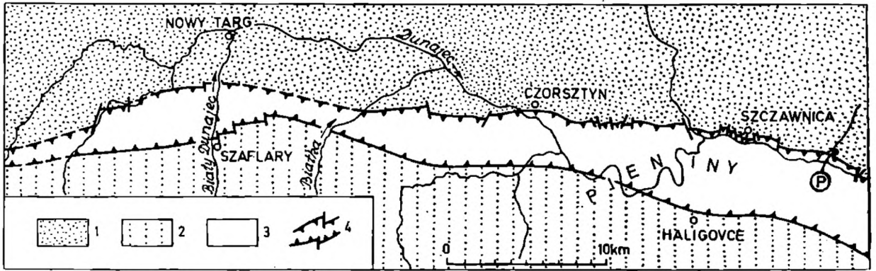
Fig. 1. Lokalizacja stanowiska z mikrofauną paleocenią (P) w Czarnej Wodzie na wschód od Szczawnicy. 1 — płaszczowina magurska; 2 — flisz podhalański; 3 — pieniński pas skałkowy; 4 — północna i południowa granica tektoniczna pienińskiego pasa skałkowego
