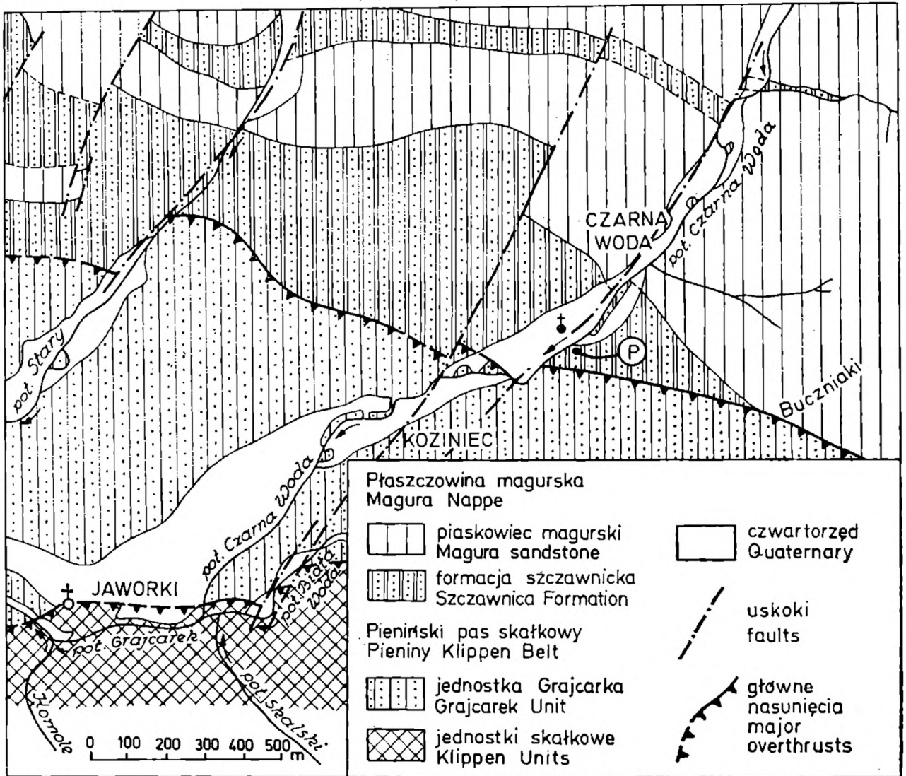
Fig. 2. Miejsce pobrania próbki z mikrofauną paleocenią (P) z formacji szczawnickiej w Czarnej Wodzie
