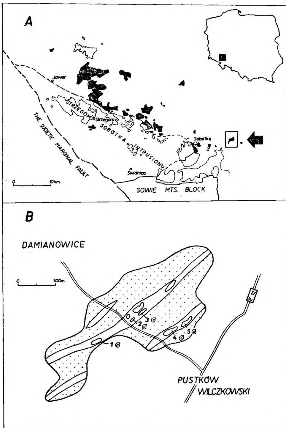
Fig. 1 A. Szkic geologiczno-tektoniczny serii metamorficznych przedpola Sudetów (na czarno zaznaczone skały metamorficzne należące do badanej serii). B. Szkic geologiczny okolic Pustkowa Wilczkowskiego (fyllity — kropki, radiolaryty — pola białe). Numerami 1—5 oznaczono stanowiska z fauną
