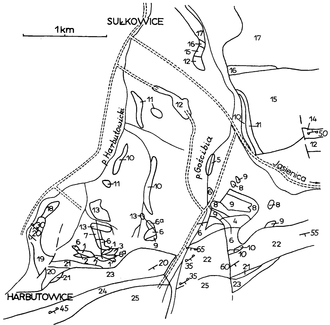
Fig. 2. Szkic geologiczny obszaru między Sułkowicami, Harbutowicami i Jasienicą. Płaszczowina podśląska: 1 — łupki wierzowskie (barem-apt), 2 — łupki lgockie (alb), 3 — łupki godulskie pstre (cenoman-turon), 4 — margle jasieniackie (cenoman-turon), 5 — margle węglowieckie (senon), 6 — łupki ciemne z piaskowcami glaukonitowymi, margle pstre, łupki ilaste pstre (paleocen-eocen dolny), 6a — zielone łupki ilaste (dolny eocen), 7 — margle szare (eocen środkowy), 8 — łupki zielone ilaste i piaskowce glaukonitowe (eocen środkowy i górny), 9 — rogowce i łupki menilitowe. Płaszczowina śląska: 10 — łupki cieszyńskie i grodziskie (walańżyn-hoteryw), 11 — łupki wierzowskie (barem-apt), 12 — warstwy lgockie (alb), 13 — warstwy barwałdzkie (alb), 14 — rogowce mikuszowickie (alb-cenoman), 15 — warstwy godulskie (cenoman-turon), 16 — pstre łupki godulskie górne (dolny senon), 17 — dolne warstwy istebniańskie (senon), 18 — rogowce i łupki menilitowe (eooligocen), 19 — warstwy krośnieńskie (oligocen). Płaszczowina magurska: 20 — piaskowiec ciężkowicki (eocen dolny), 21 — łupki pstre w różnych poziomach eocenu dolnego i środkowego, 22 — piaskowiec pasierbiecki dolny (eocen środkowy), 23 — piaskowiec pasierbiecki górny (eocen środkowy), 24 — warstwy podmagurskie (eocen górny), 25 — piaskowiec magurski (eocen górny-oligocen)
