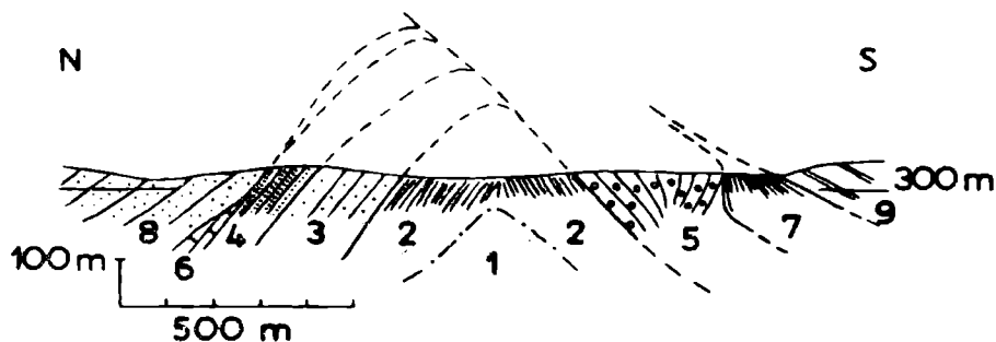
Fig. 1. Przekrój przez strefę lanckorońską w Barwałdzie Średnim Płaszczyzna podśląska: 1 — warstwy gezowe; płaszczyzna śląska: 2 — łupki wierzowskie, 3 — warstwy lgockie dolne, 4 — warstwy lgockie środkowe, 5 — warstwy barwałdzkie, 6 — warstwy lgockie górne (rogowce mikuszowickie), 7 — pstre łupki godulskie, 8 — warstwy istebniańskie, 9 — warstwy krosnieńskie
