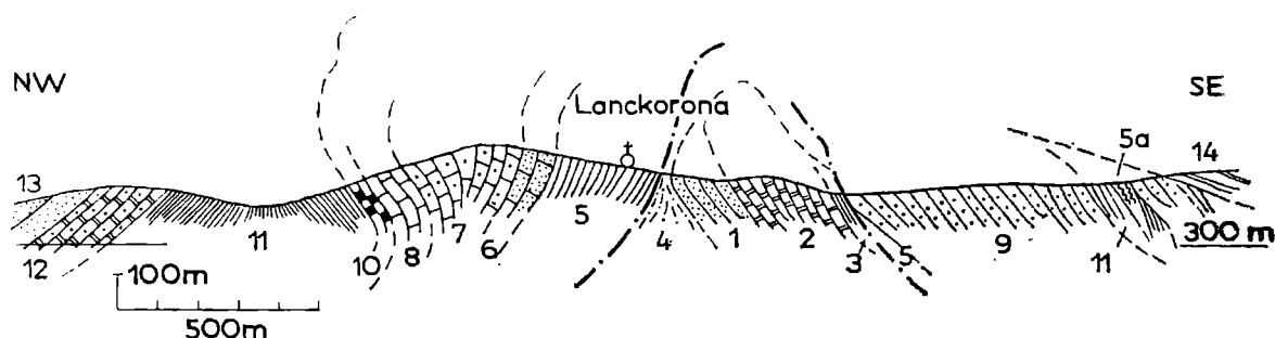
Fig. 4. Przekrój strefy lanckorońskiej w Lanckoronie. Płaszczowina podśląska: 1 — piaskowce grodziskie (ostrygowe) (górny barem-dolny apt), 2 — warstwy gezowe (alb), 3 — pstre łupki godulskie (cenoman-turon), 4 — margle pstre węglowieckie (senon). Płaszczowina śląska: 5a — łupki cieszyńskie górne (walanżyn), 5 — łupki wierzowskie (barem-dolny apt), 6 — warstwy lgockie dolne, 7 — warstwy lgockie środkowe (6-7 — alb), 8 — warstwy lgockie górne (rogowce mikuszowickie, alb-cenoman), 9 — warstwy barwałdzkie (alb), 10 — radiolaryty, 11 — pstre łupki godulskie (10-11 — cenoman-turon), 12 — warstwy godulskie (turon), 13 — warstwy istebniańskie dolne (senon), 14 — warstwy krośnieńskie (oligocen)
