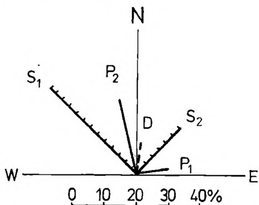
Fig. 5. Schemat kierunków spękań i szczelin w skałach permu monokliny przedsudeckiej, objaśnienia w tekście Fig. 5. Scheme of directions of joints and fractures in Permian rocks of the Fore-Sudetic Monocline; explanations in the text
