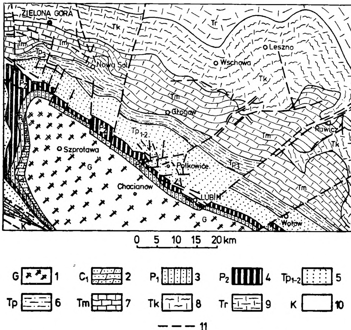
Fig. 1. Wycinek odkrytej mapy geologicznej monokliny przedsudeckiej wg J. Sokołowskiego, nieco uproszczony. 1 — prekambry i starszy paleozoik bloku przedsudeckiego; 2 — dolny karbon; 3 — czerwony spągowiec; 4 — cechsztyń; 5 — dolny i środkowy pstry piaskowiec; 6 — górny pstry piaskowiec (ret); 7 — wapień muszlowy; 8 — kajper; 9 — retyk; 10 — górna kreda; 11 — uskoki
