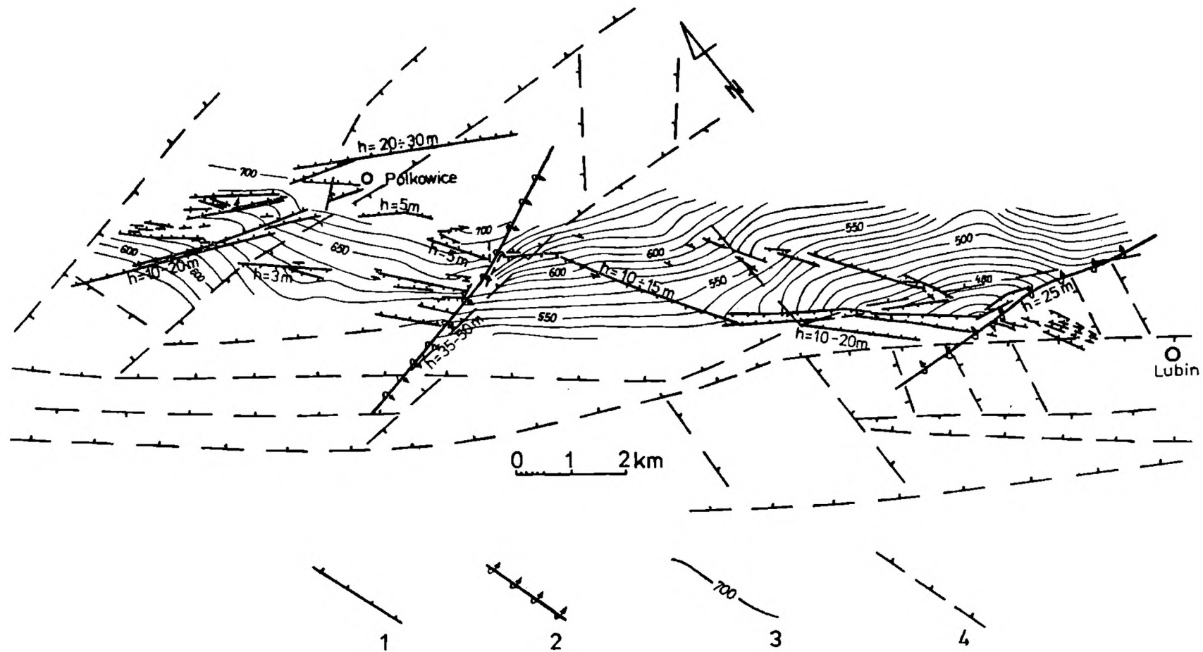
Fig. 4. Szkic tektoniczny obszaru miedzionośnego rozpoznanego wyrobiskami górnictwymi. 1 — uskoki normalne; 2 — uskoki inwersyjne; 3 — izoliny spągu serii wapienno-dolomitowej cechsztynu; 4 — uskoki przewidywane w dokumentacji geologicznej na podstawie rozpoznania otworami wiertniczymi
