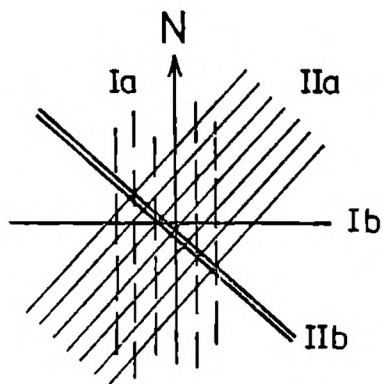
Fig. 2. Orientacja osi fałdków ciągniętych i rys ślizgowych w łupkach miedzionośnych. I — rysy ślizgowe o przebiegu N-S (Ia) związane genetycznie z osiami fałdków ciągniętych o przebiegu W-E (Ib); II — rysy ślizgowe o przebiegu NE-SW (IIa) związane genetycznie z osiami fałdków ciągniętych o przebiegu NW-SE (IIb)
