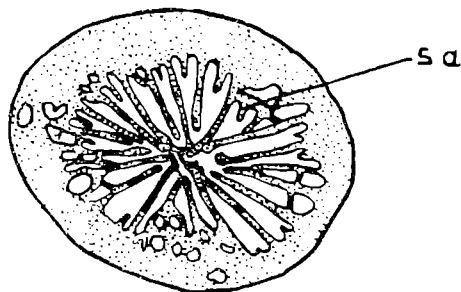
Fig. 4. Procladocora sp., coupe transversale du polypiérite, \times 3 , s a — septe abortif
