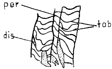
Fig. 3. Diplotheophyllia aff. basseae All., coupe longitudinale de deux polypiérites et d'un fragment de périthèque, X 4. t — planchers, dis — dissépiments, per — périthèque
