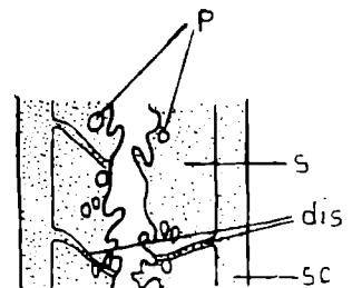
Fig. 5. Calamophylliopsis fotisalensis (Bendukidze), fragment d'une coupe transversale d'un polypiérite, \times 7 .
