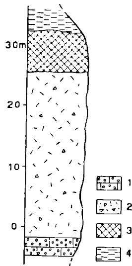
Fig. 2. Profil de l'Urgonien de la série haut-tatrique au-dessous de Giewont (simplifié). Pour explication des symboles voir Fig. 1
