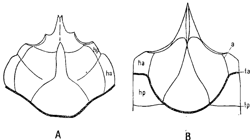
Fig. 2. Homologies probables des sillons de Laeviprosopon laeve (A) et Gastrosacus wetzleri (B). Le trait épais marque le sillon cervical tel qu'il est désigné chez les deux formes. On voit que seules les parties médianes en sont homologues. Les parties latérales du sillon cervical de L. laeve correspondent aux sillons transversaux postérieurs de Gastrosacus wetzleri ; ha — régions hépatiques antérieures; hp — régions hépatiques postérieures
