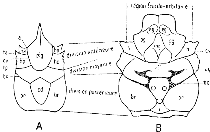
Fig. 1. Division du céphalothorax chez les Galatheïdés: Munidopsis antonii (A) et des Dromiacés: Prosopon verrucosum (B); plg — plastron gastrique, eg — régions épigastriques; mg — région mésogastrique; pg — régions paragastriques; h — régions hépatiques antérieures (ha), postérieures (hp); ugs — région urogastrique, cd — région cardiaque; br — régions branchiales; i — région intestinale; cv — sillon cervical; ug — sillon urogénital; bc — sillon branchiocardiaque; a — sillon antennaire; ta — sillon transversal antérieur ou hépatique; tp — sillon transversal postérieur ou branchiohépatique
