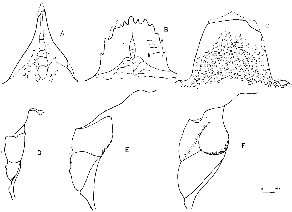
Fig. 3. Rostre de: A — Gastrosacus eminens (Blaschke) Tithonique de Sinaïa; B — Galathea (Palaeomunida) n. sp. (Tithonique de Purcăreni); C — Galathea (Paragalathea) verrucosa Moericke (Tithonique de Moroeni); région ptérygostomiale de D — Longodromites angustus (Reuss) (Tithonique de Sinaïa); E — Pithonoton etalloni (G. G. Gemmellaro) (Tithonique de Sinaïa); F — Eodromites grandis (Meyer) (Tithonique de Sinaïa)
