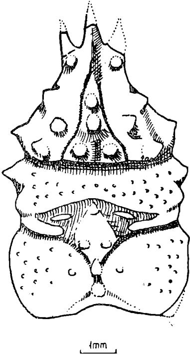
Fig. 5. Nodoprosopon ornatum carpaticum n. subsp. Patrulius, du Tithonique inférieur de Woźniki
