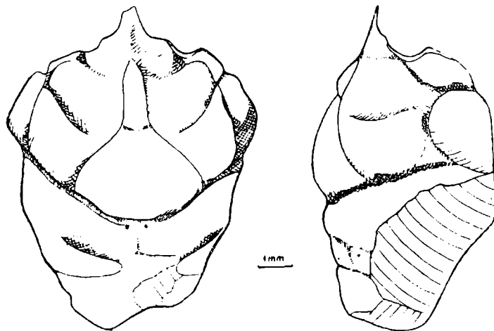
Fig. 4. Laeviprosopon laeve (Meyer), du Tithonique inférieur de Woźniki
