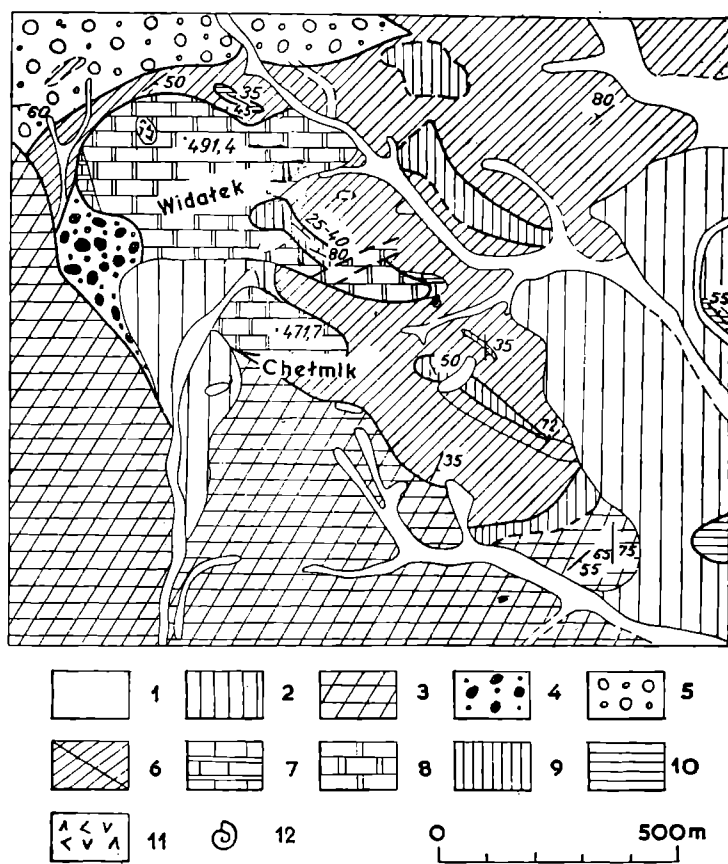
Fig. 1. Szkic geologiczny wzgórza Chełmik, na podstawie nie publikowanego zdjęcia geologicznego J. Oberca. Arkusz Nowa Ruda, Holocen; 1 — aluwia; plejstocen: 2 — gliny; czerwony spągowiec: 3 — zlepieńce, piaskowce, łupki; górny karbon: 4 — warstwy białokamięskie, facja noworudzka; dolny karbon: 5 — zlepienie z Wilczy; 6 — łupki i szarogłazy kulmu; 7 — wapień węglowy; 8 — karbon Widałka—Chełmika, dolny dewon: 9 — warstwy z Wilczy; 10 — łupki zdanowskie, 11 — gabbro; 12 — stanowisko z fauną
