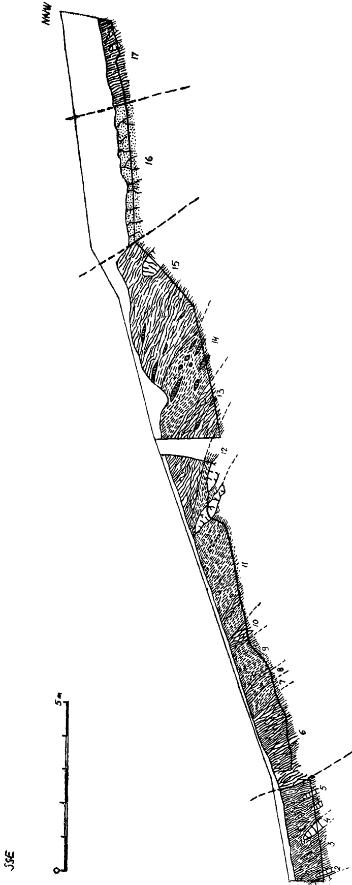
Fig. 1. Profil geologiczny (nr 32) sztucznego odsłonięcia na wzgórzu Wronine koło zamku czorsztyńskiego. Objasnienia w tekście. Grubsze linie oznaczają najważniejsze kontakty tektoniczne.
