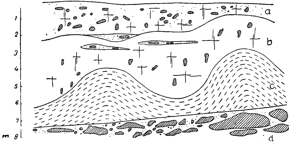
Fig. 1. Przekrój geologiczny osadów czwartorzędowych w cegielni jeleniogórskiej. a — glina morenowa piaszczysta barwy brązowej; b — glina morenowa ilasta, barwy ciemnoszarej; c — łą warwowe; d — osad typu proluwialnego
