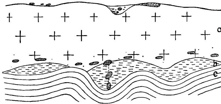
Fig. 4. Sposób subglacjalnej sedymantacji materiału skalnego. a — lód; b — woda; c — il warwowy
