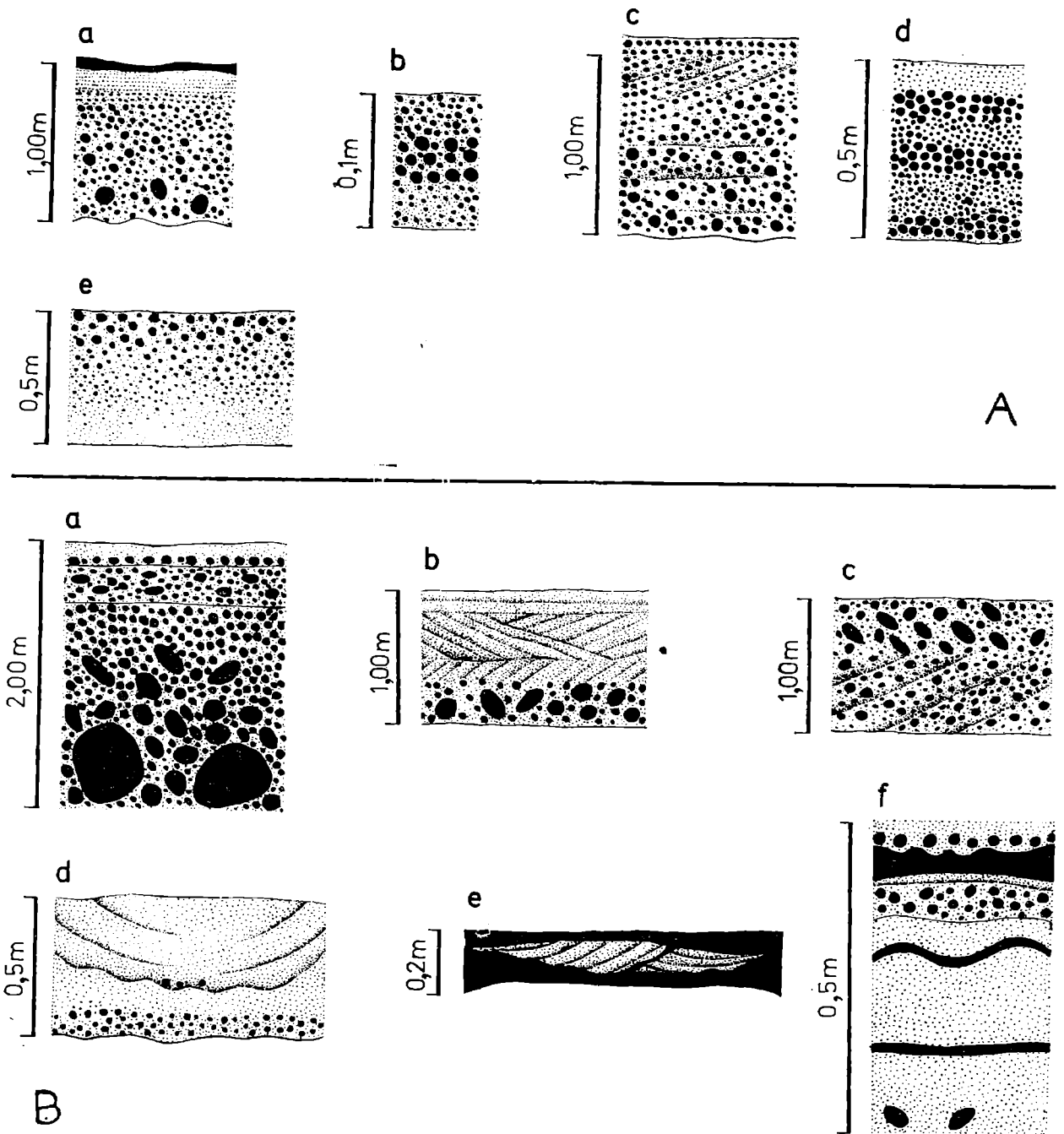
Fig. 14. Types of bedding in the Lower (A) and Upper (B) Świerzawa Member Fig. 14. Typy warstwowań w dolnej (A) i górnej (B) serii świerzawskiej
