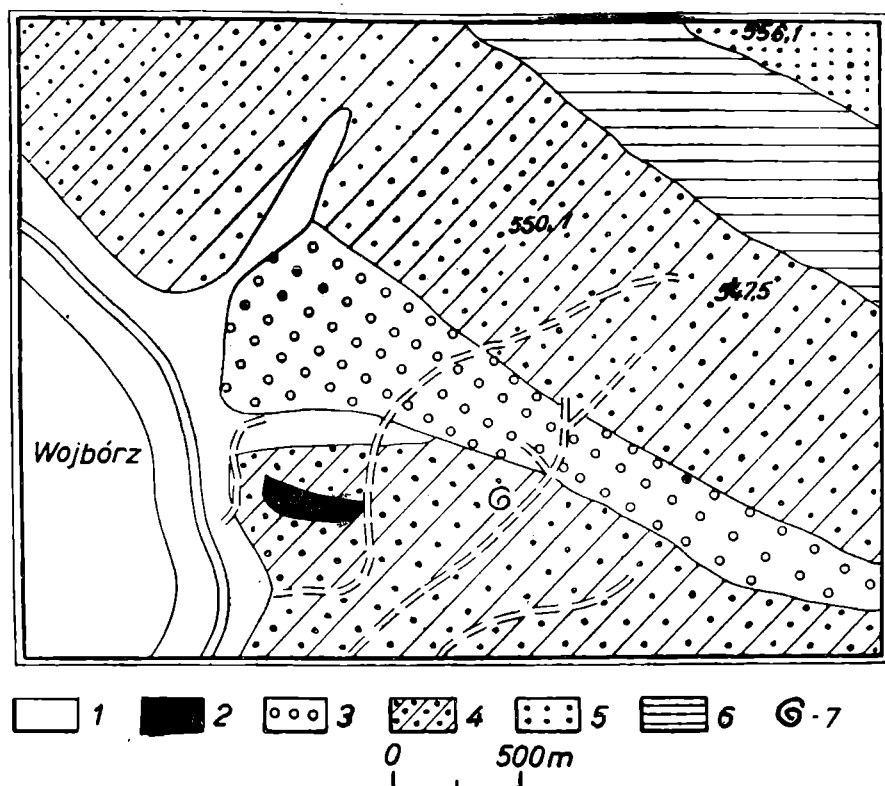
Fig. 1. Szkic sytuacyjny stanowiska z fauną (geologia wg. J. Oberca). 1 — aluwia; 2 — kersantyt; dolny karbon; 3 — zlepieniec z Wilczy; 4 — seria łupkowo-szarogłazowa; 5 — szarogłazy; 6 — dewon; 7 — stanowiska z fauną
