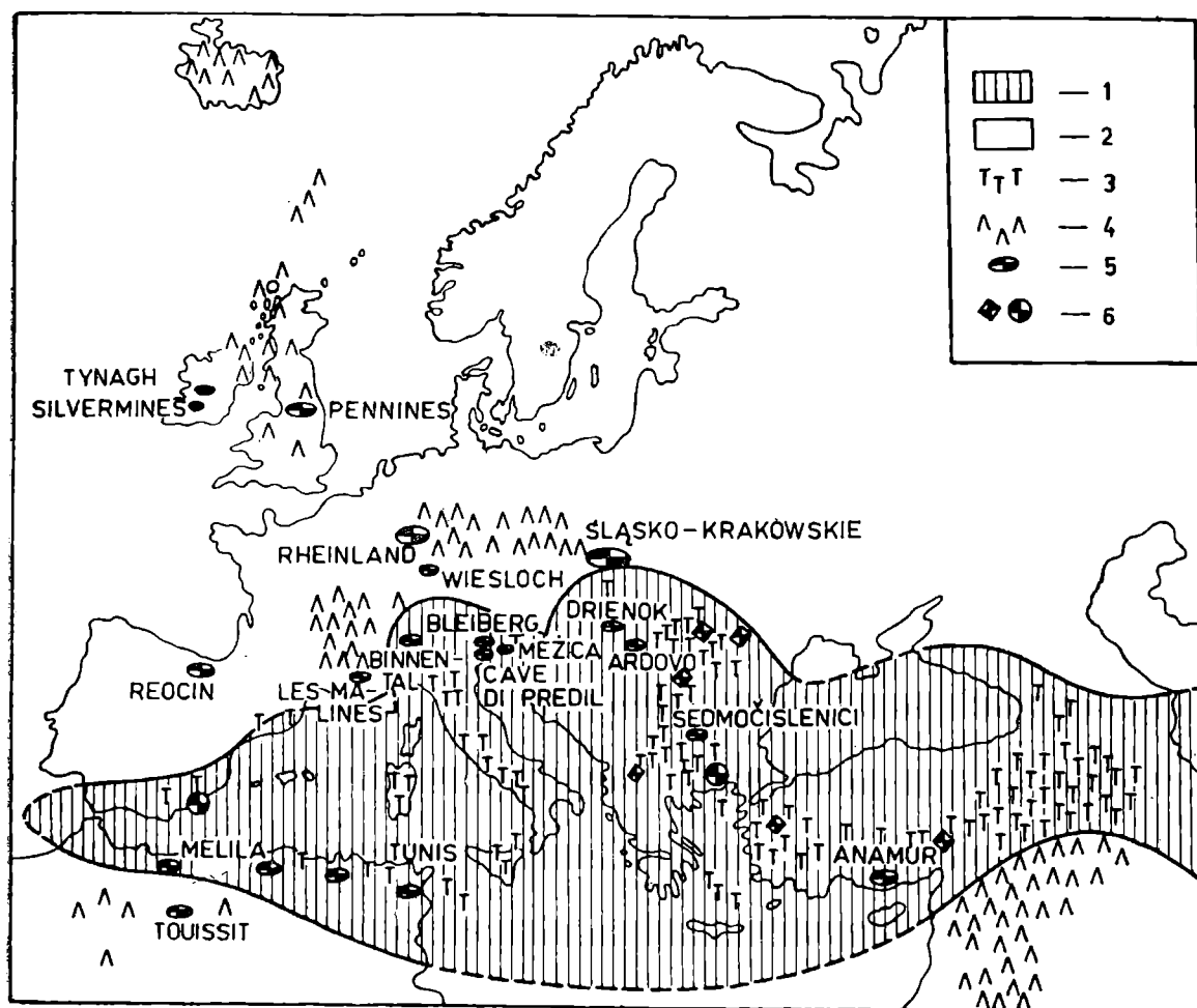
Fig. 2. Sytuacja metalogeniczna złóż Zn-Pb (szczególnie typu S-C) powstałych w końcu cyklu alpejskiego w Europie. 1 — strefa mobilna (geosynklina); 2 — strefa stabilna (platforma); 3 — magmatyzm stadium końcowego strefy mobilnej; 4 — równoległy magmatyzm strefy stabilnej; 5 — złoża Zn-Pb typu S-C; 6 — inne złoża Zn-Pb Fig. 2. Metallogenic situation of the lead-zinc deposits (particularly of the Silesian-Cracovian type) formed during the final stage of the Alpine cycle in Europe. 1 — mobile zone (geosyncline); 2 — stable zone (platform); 3 — magmatism of the final stage in the mobile zone; 4 — simultaneous magmatism of the stable zone; 5 — zinc-lead deposits of the Silesian-Cracovian type; 6 — another Zn-Pb deposits
