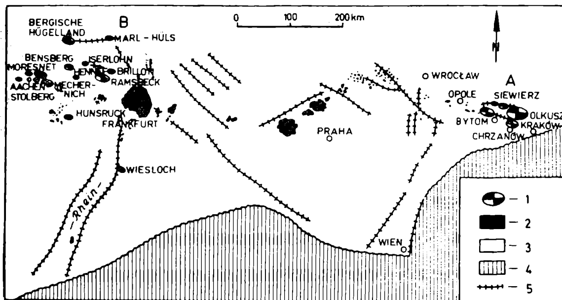
Fig. 1. Pozycja złóż śląsko-krakowskich i Nadrenii. A — złoża śląsko-krakowskie; B — złoża Nadrenii; 1 — złoża cynkowo-ołowiowe typu S-C (Silesian-Cracovian); 2 — neogeńskie skały magmowe zasadowo-alkaliczne; 3 — strefa stabilna (platforma) w cyklu alpejskim; 4 — strefa mobilna (geosynklina) w cyklu alpejskim; 5 — duże zaburzenia geotektoniczne (głównie dyslokacje), przeważnie trzeciorzędowe
