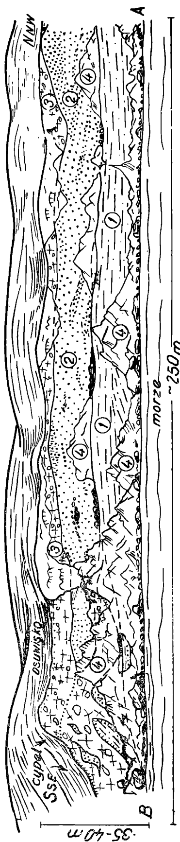
Fig. 2. Fragment południowej części klifu redłowskiego (rysunek wykonany w kwietniu — maju 1958). 1 — utwory miocenijskie; 2 — fluwiogłacjat; 3 — gliny zwałowe; 4 — obsunięcia, zwaliska, osypiska (zaznaczono dla przejrzystości częściowo)
