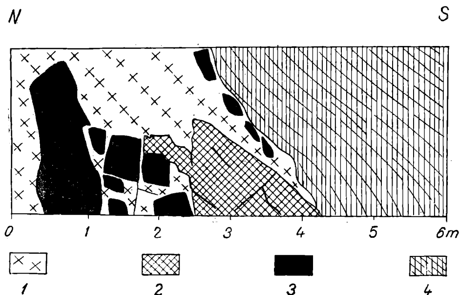
Fig. 1. Bryły soli dolomitycznej w zubrze (poziom kopalniany III, chodnik „Kaniów”.) 1 — Druzgot iłowo-solny (zuber); 2 — porwak soli kamiennej dolomityczno-kalcytowej; 3 — bryły iłowca marglistego (mydlarka); 4 — sól kamienna ilasta, warstwowana, tzw. „spizowa”.
