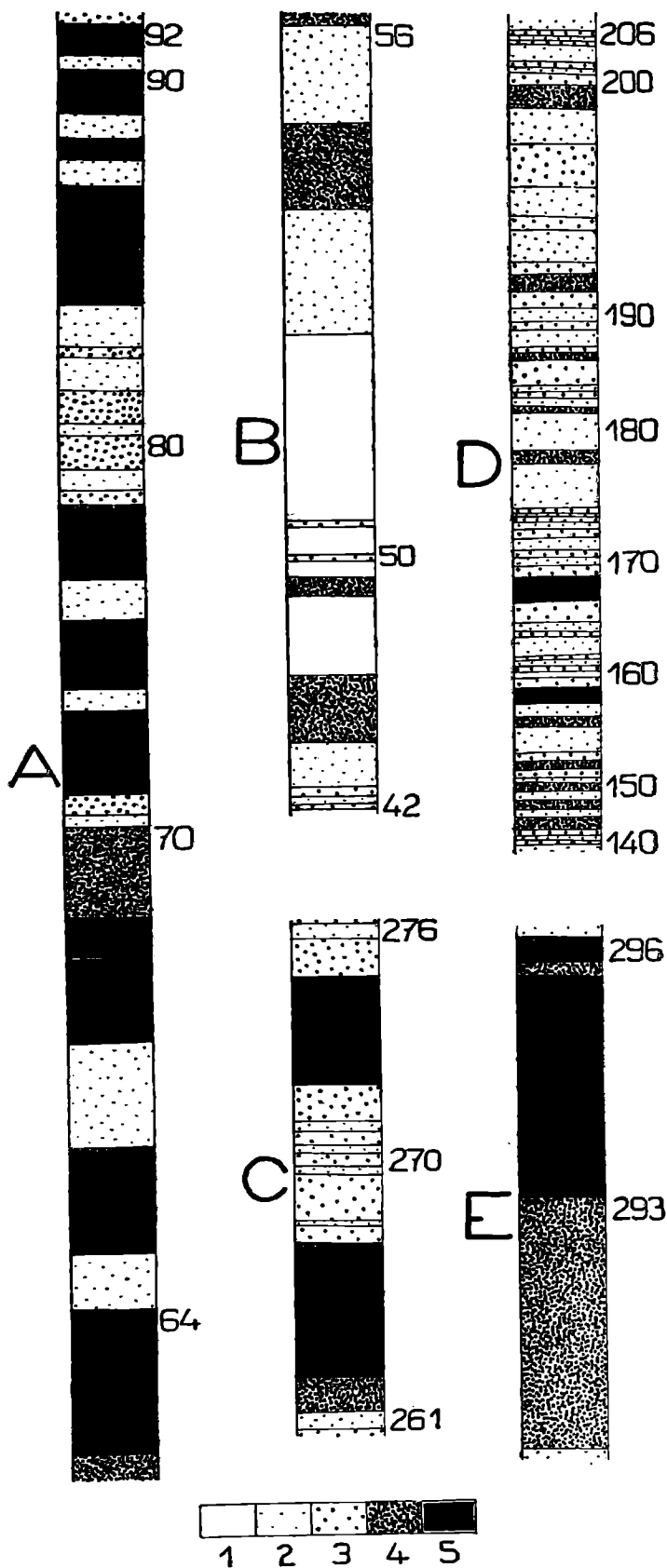
Fig. 2. Charakterystyczne kompleksy warstw odrysowane z profilu wykonanego w podziałce naturalnej. Objaśnienie znaków: 1=iłły, 2=piaski ilaste 3=piaski drobne, 4=piaski gruboziarniste, 5=żwirry. Liczby oznaczają numerację warstw. — A=żwirry i piaski dolnej części ozu. B=wkładka iłów w dolnej części ozu, C=różnica miąższości warstw letnich i zimowych, D=warstwy z środkowej części ozu, E=żwirry i piaski gruboziarniste z górnej części ozu.
