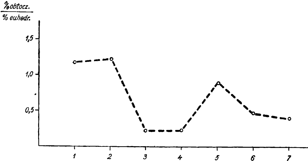
Fig. 1. Diagram stosunku występowania ziarn cyrkonu anhidralnych obtoczonych i euhedralnych w piaskowcach egzotycznych z Bachowic:
